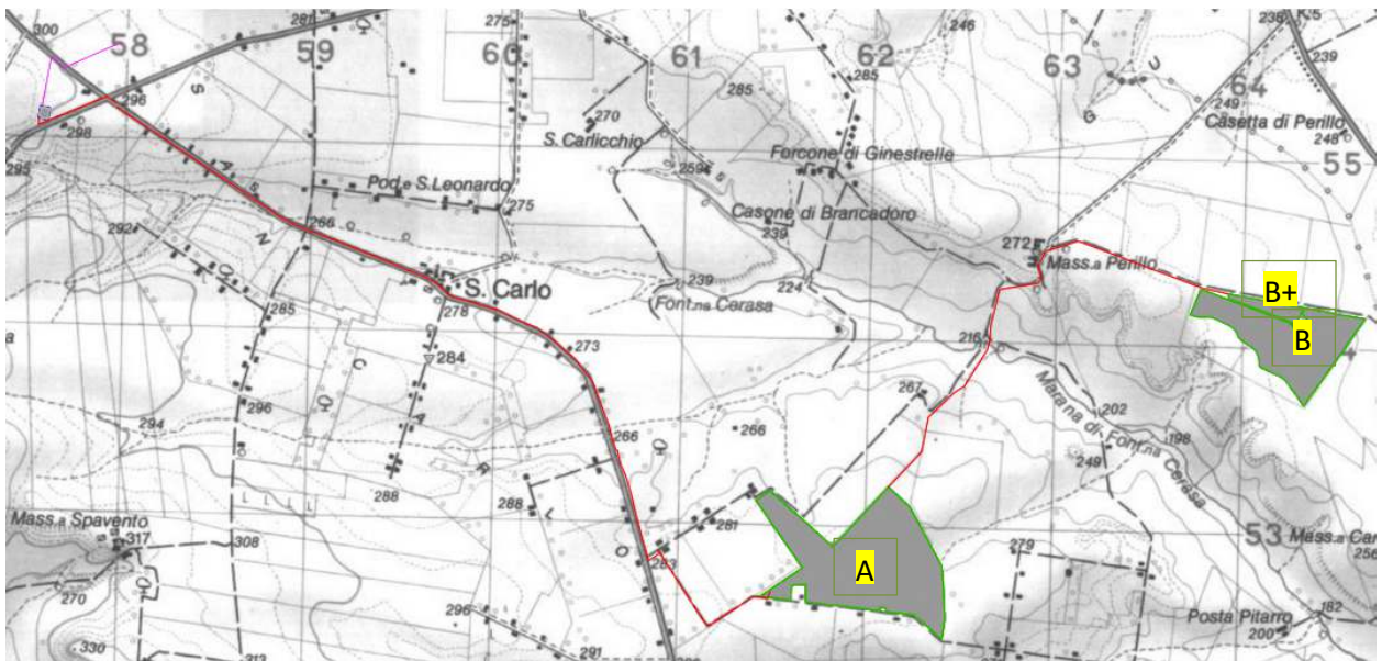
Fig. 3 ubicazione impianto fotovoltaico e opere di connessione
