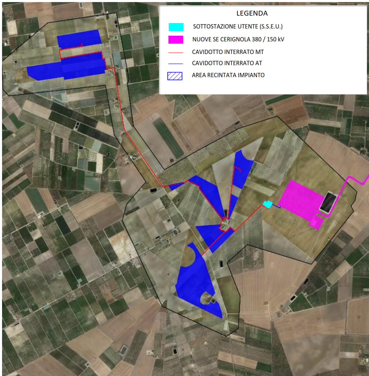
Fig. 2 Inquadramento territoriale opere di connessione su ortofoto
