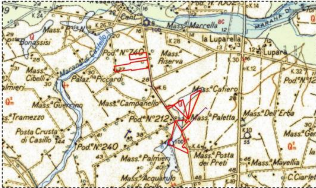
Stralcio Carta Geologica d'Italia 1:100.000, Foglio 164 "Foggia"
