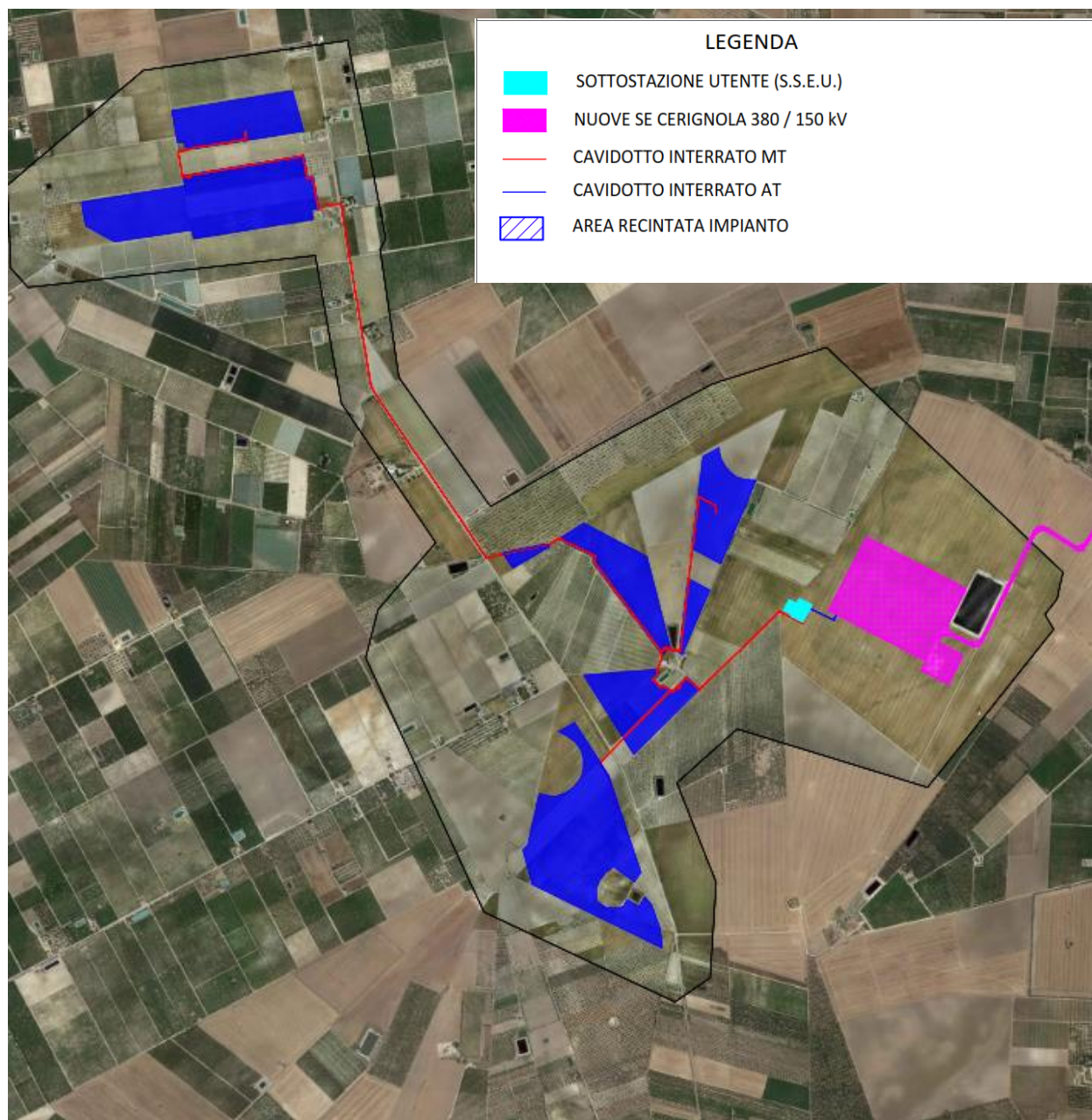
Fig. 5 Ortofoto ubicazione opere di connessione
