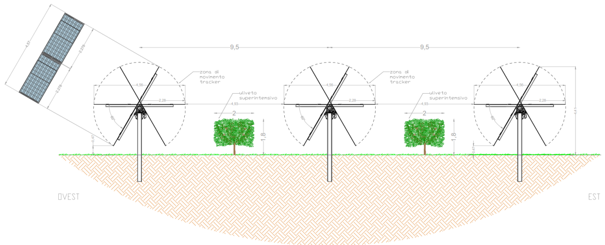
Fig. n°19 Pitch dei tracker
