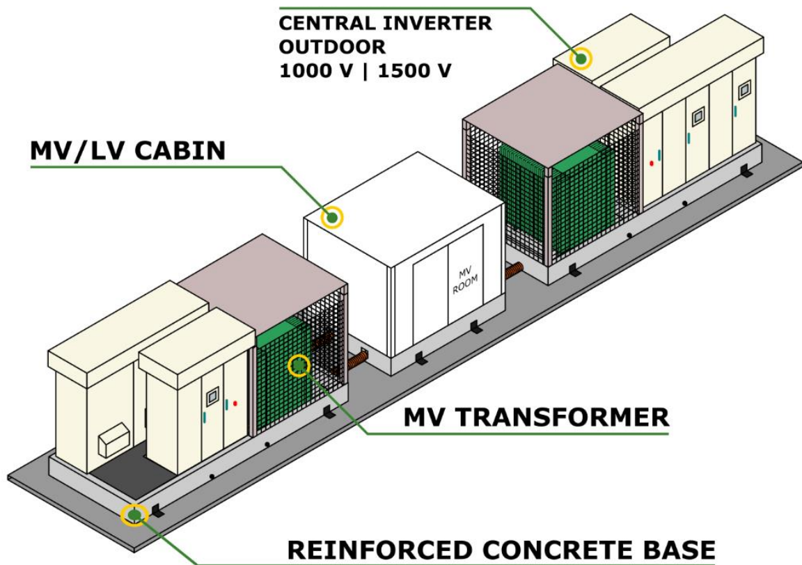
Fig. n°16 Power Skid
