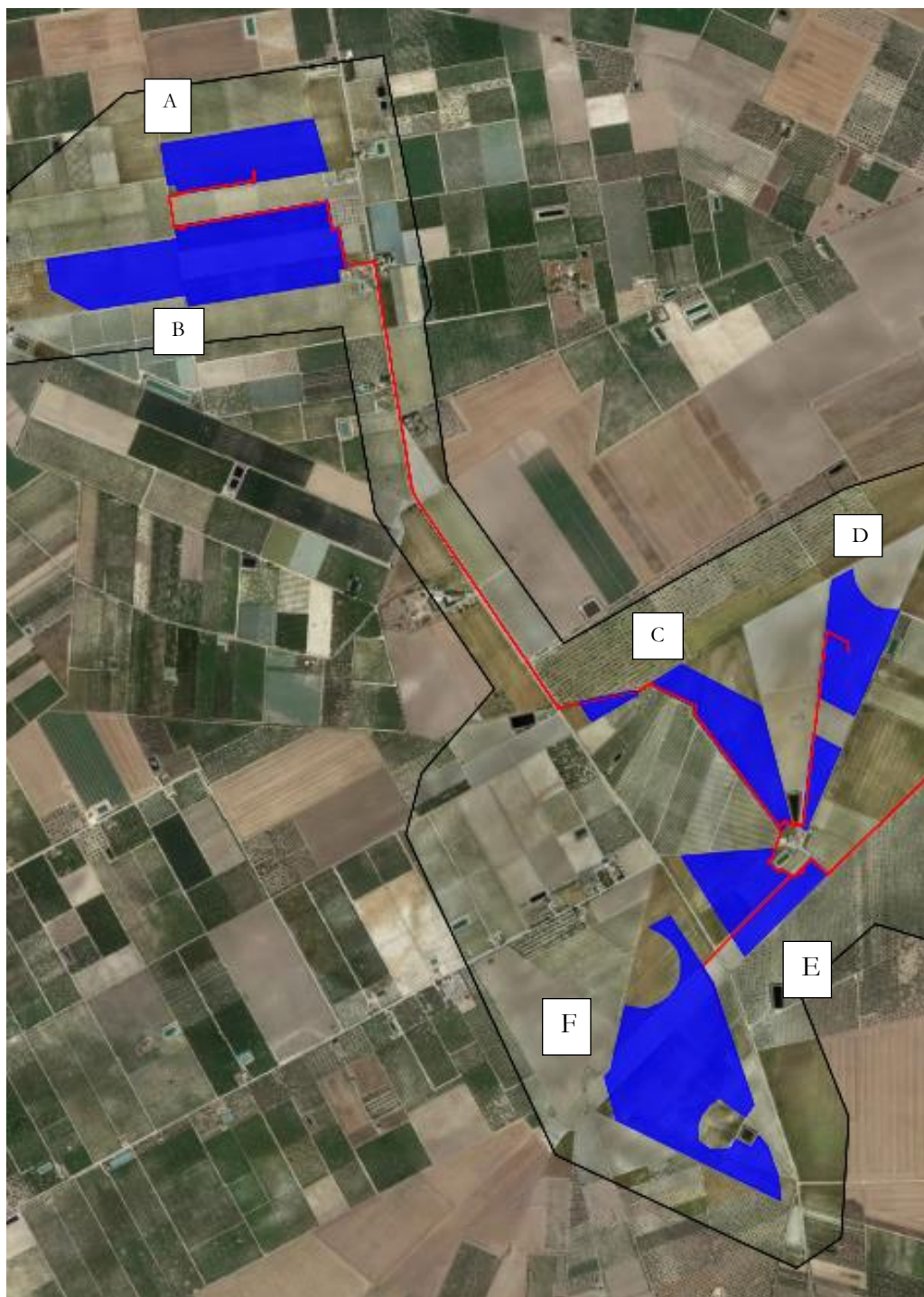
Fig. n°2 Inquadramento su ortofoto dell'impianto agro-fotovoltaico e delle opere di connessione
