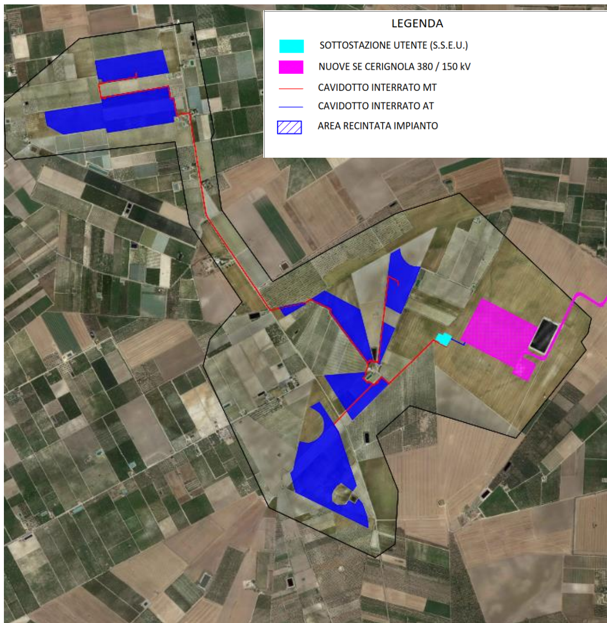
Fig. 7 Inquadramento territoriale opere di connessione su ortofoto
