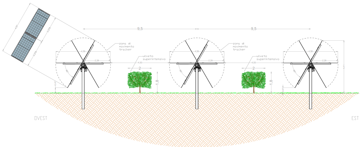
Fig. n°1 Sistema Agro-fotovoltaico
