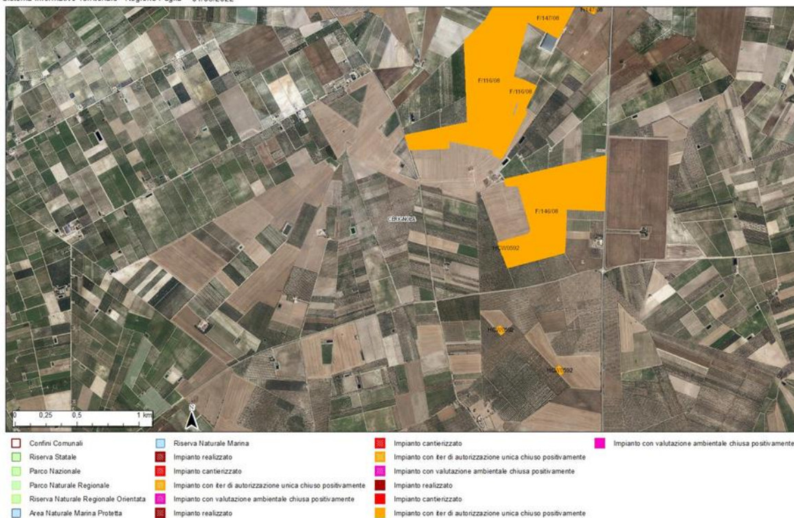
Figura 1-23: Impianti nell'Area di Visibilità Teorica – Particolare sud – Fonte SIT Puglia
