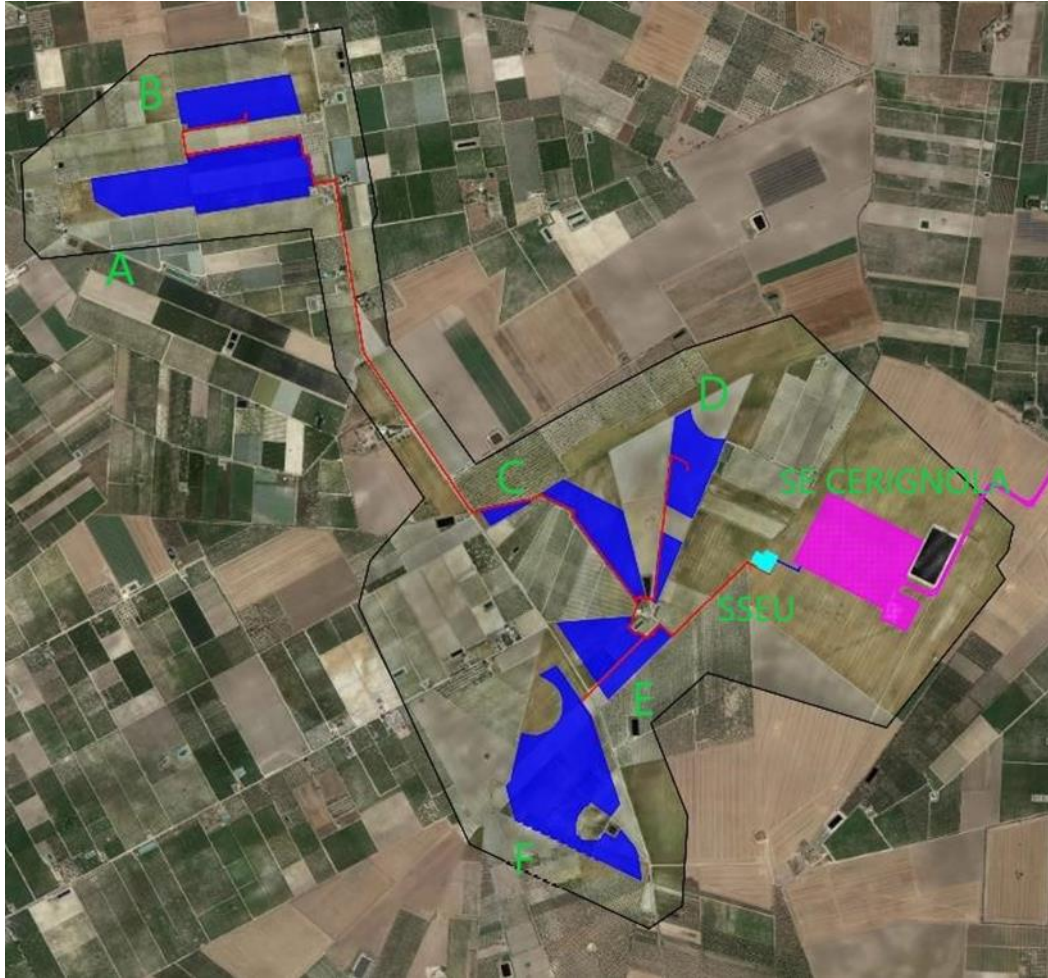
Figura 1-4: Inserimento dell'impianto nel contesto circostante a carattere agricolo principale
