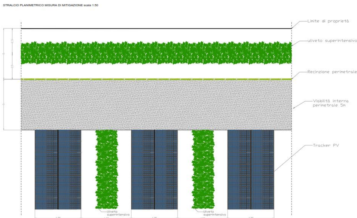
Figura 1-2: Schema esempio d'impianto uliveto super intensivo tra i pannelli fotovoltaici
