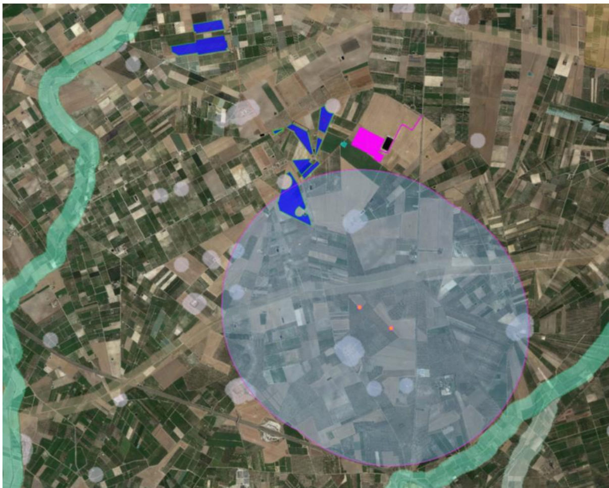
Figura 1-28: Individuazione degli impianti eolici presenti nell'area del dominio – Autorizzati ma non realizzati.
