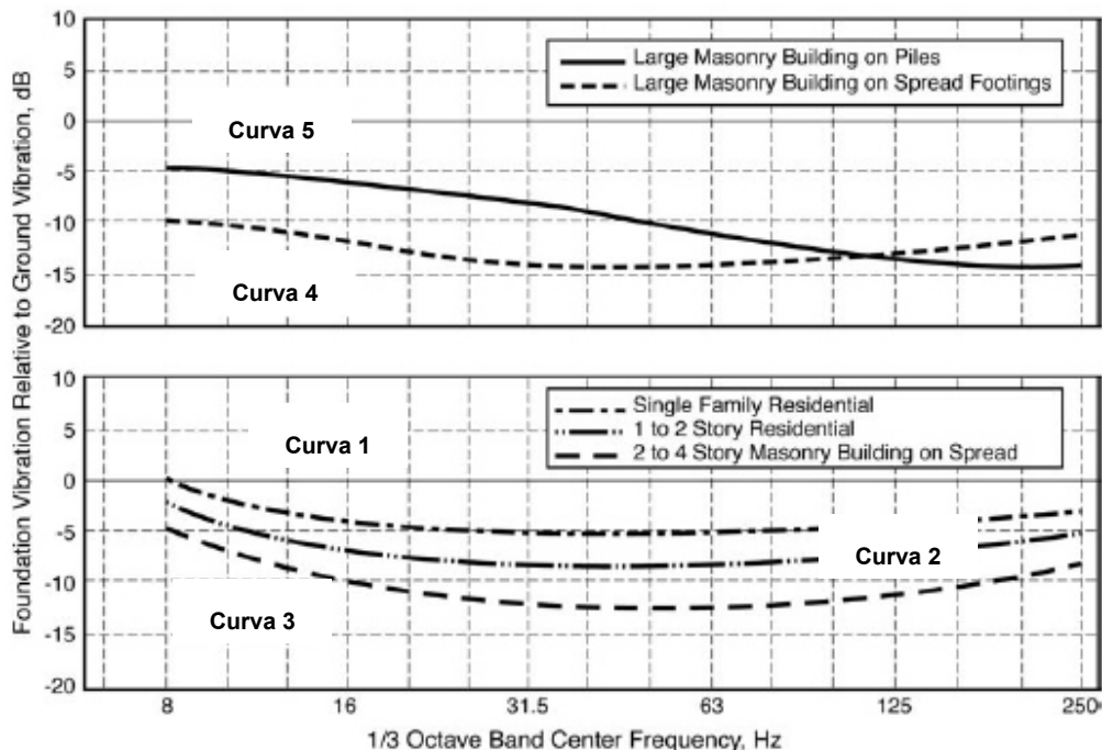
Figura 5-13 Fattori correttivi dovuti alla tipologia di fondazione
