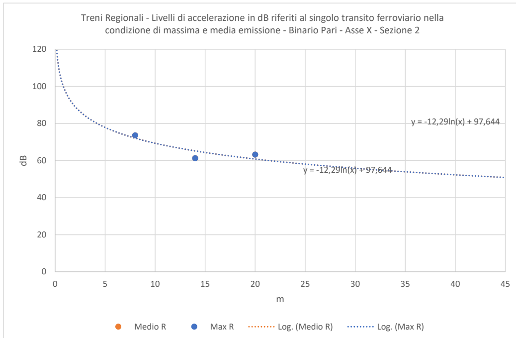
Figura 5-8 Individuazione della legge di propagazione delle vibrazioni nel terreno sulla base dei dati sperimentali lungo l'asse Y per la tipologia di treno regionale nella condizione di massima e media emissione.
