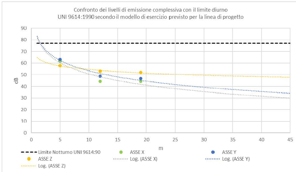
Figura 6-2 Confronto dei livelli di emissione complessiva all'interno degli edifici con i limiti UNI 9614:1990 in funzione della distanza dal binario secondo il modello di esercizio previsto – Periodo diurno.
