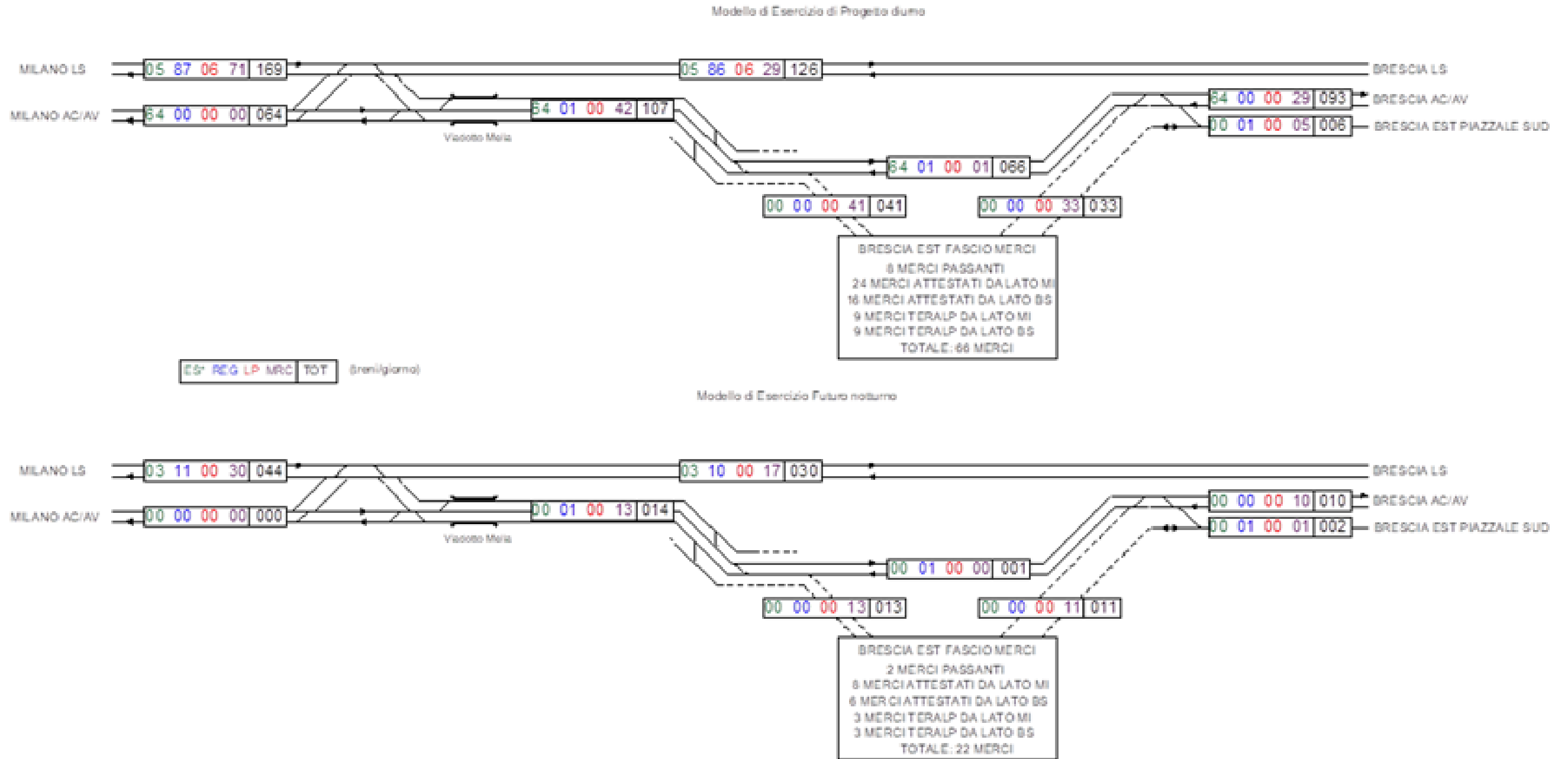
Figura 6-1 - Indicazione schematica delle tratte di intervento in progetto con indicazione dei traffici ferroviari.
