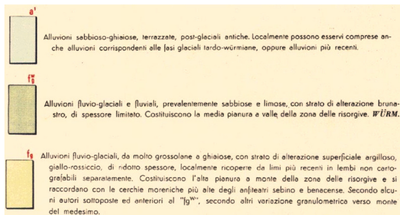
Figura 3-2 Stralcio non in scala della Carta Geolitologica d'Italia in scala 1:100.000.
