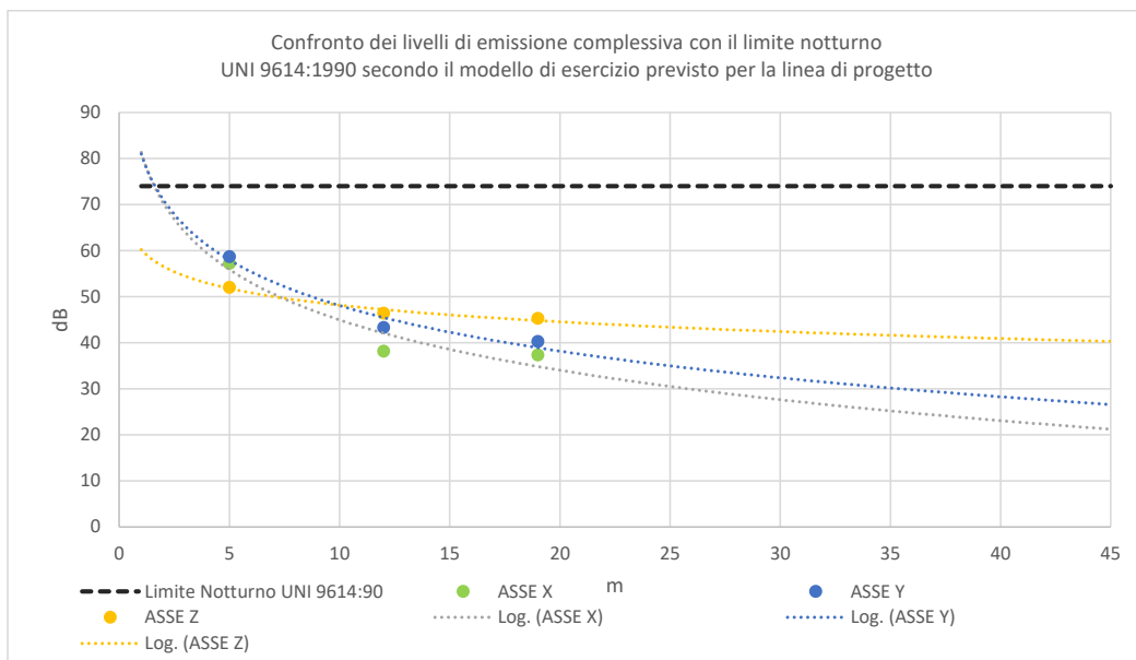
Figura 6-3 Confronto dei livelli di emissione complessiva all'interno degli edifici con i limiti UNI 9614:1990 in funzione della distanza dal binario secondo il modello di esercizio previsto – Periodo notturno, tratta M.
