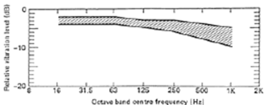
Figura 5-11 Attenuazione delle vibrazioni nel passaggio da un piano al successivo
