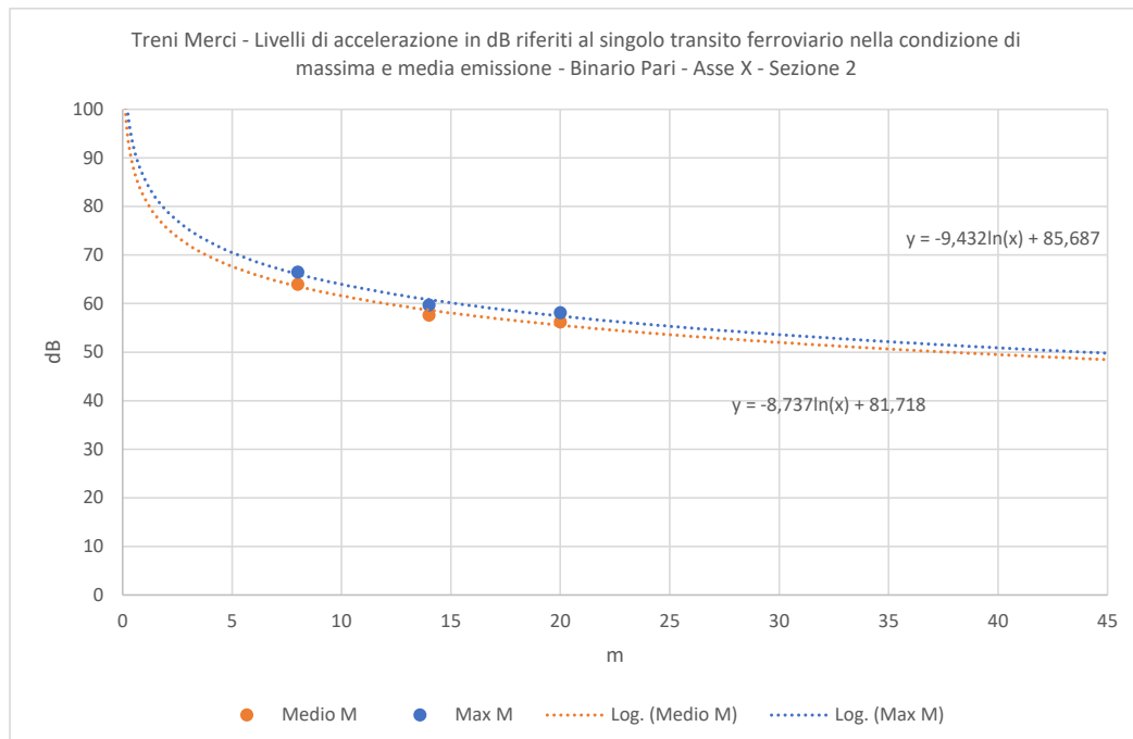
Figura 5-6 Individuazione della legge di propagazione delle vibrazioni nel terreno sulla base dei dati sperimentali lungo l'asse Z per la tipologia di treno mercè nella condizione di massima e media emissione.
