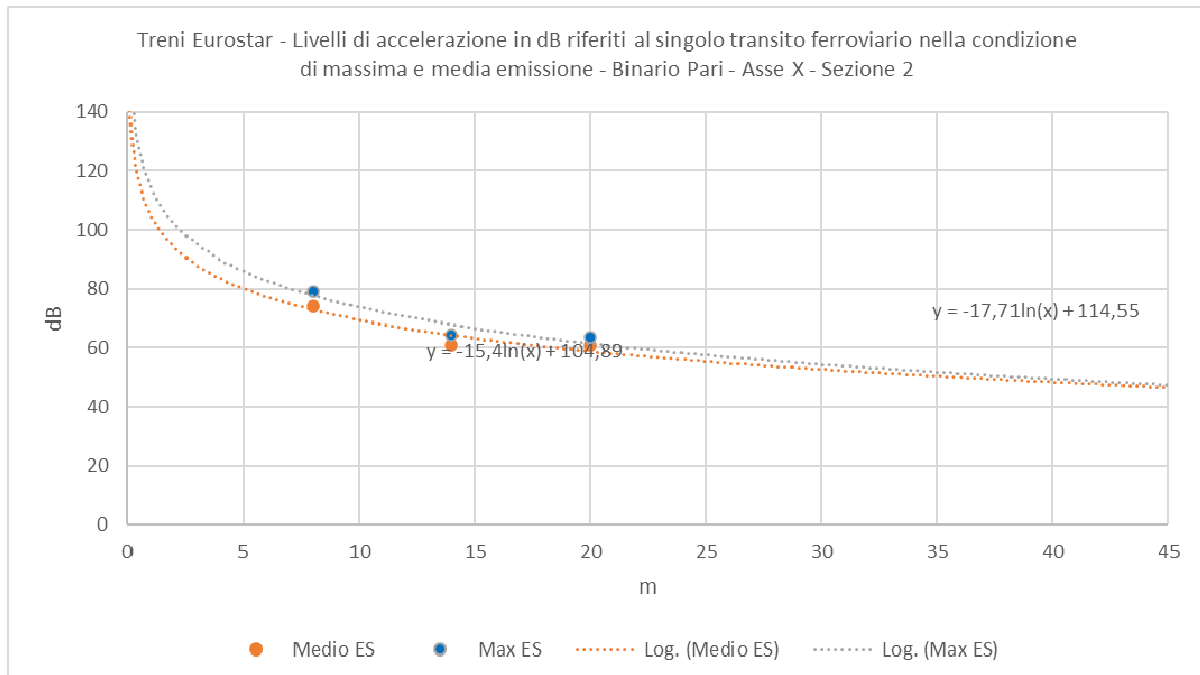
Figura 5-2 Individuazione della legge di propagazione delle vibrazioni nel terreno sulla base dei dati sperimentali lungo l'asse Y per la tipologia di treno Eurostar nella condizione di massima e media emissione.
