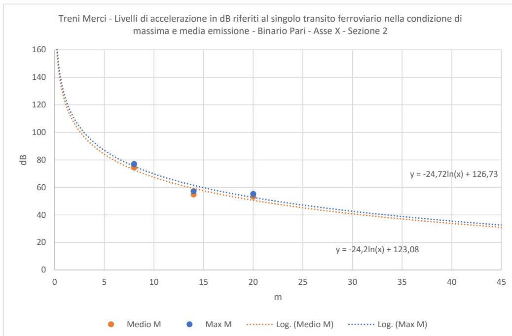
Figura 5-4 Individuazione della legge di propagazione delle vibrazioni nel terreno sulla base dei dati sperimentali lungo l'asse X per la tipologia di treno mercì nella condizione di massima e media emissione.
