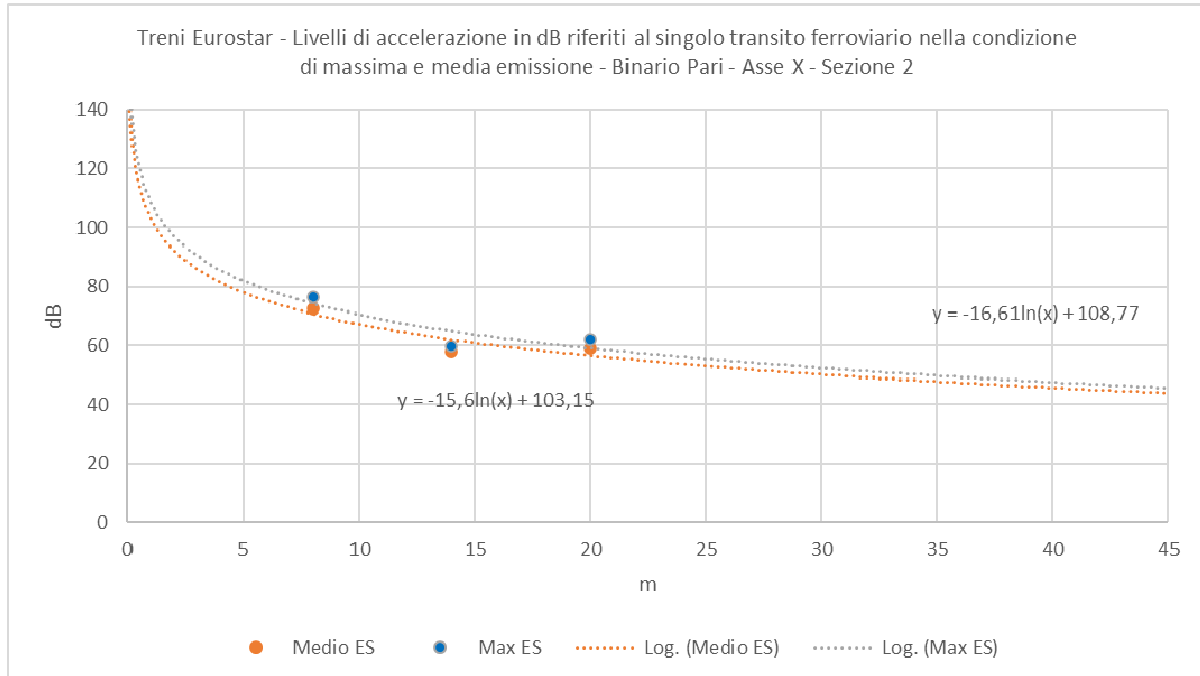
Figura 5-1 Individuazione della legge di propagazione delle vibrazioni nel terreno sulla base dei dati sperimentali lungo l'asse X per la tipologia di treno Eurostar nella condizione di massima e media emissione.
