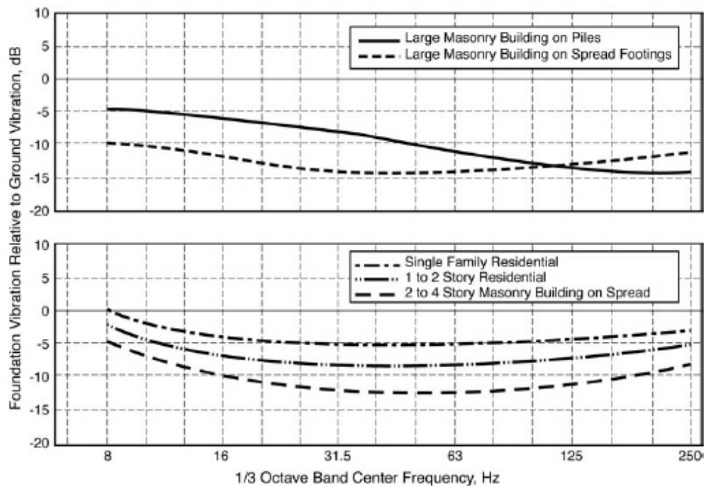
Figura 5-10 Risposta delle fondazioni per diverse tipologie di edifici (Fonte: FTA, USA)
