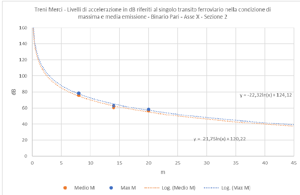
Figura 5-5 Individuazione della legge di propagazione delle vibrazioni nel terreno sulla base dei dati sperimentali lungo l'asse Y per la tipologia di treno mercè nella condizione di massima e media emissione.
