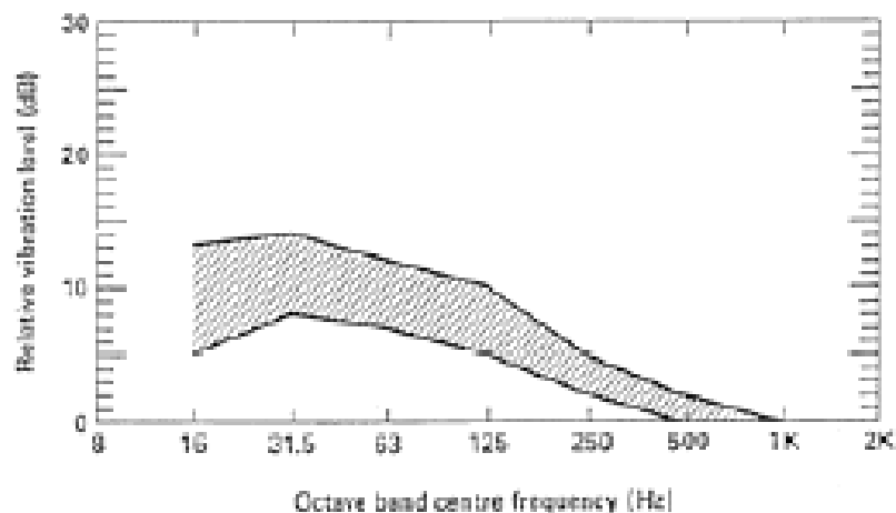
Figura 5-12 Amplificazione prodotta dai solai
