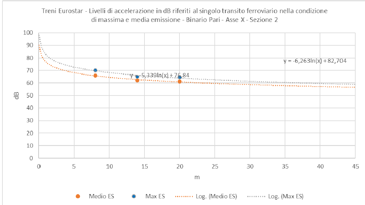
Figura 5-3 Individuazione della legge di propagazione delle vibrazioni nel terreno sulla base dei dati sperimentali lungo l'asse Z per la tipologia di treno Eurostar nella condizione di massima e media emissione.
