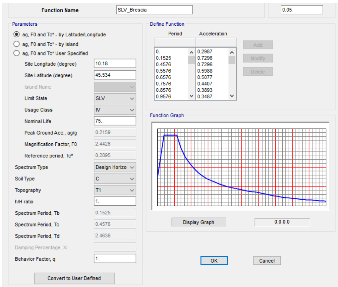
Figura 6-4 – Spettro di risposta definito all'interno di SAP2000 allo SLV
