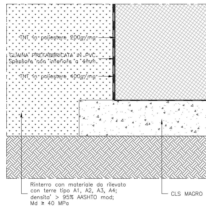
PARTICOLARE "Y" SCALA 1:10
