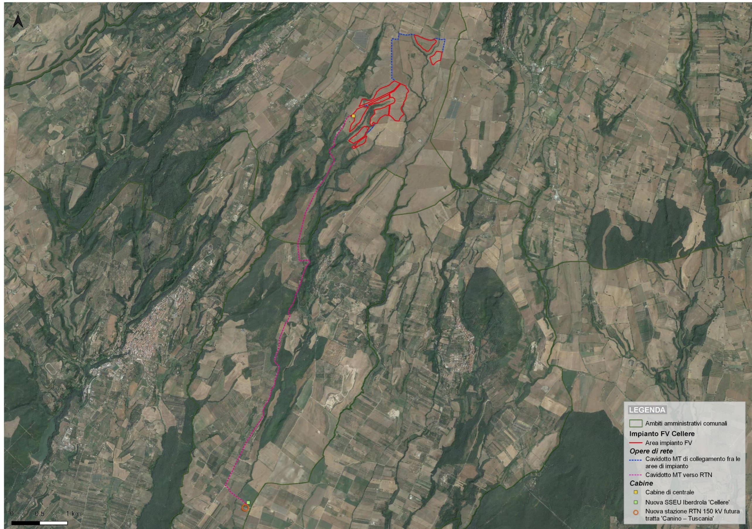
Figura 1 – Ortofoto con progetto (impianto FV, cavidotto interrato e cabine)
