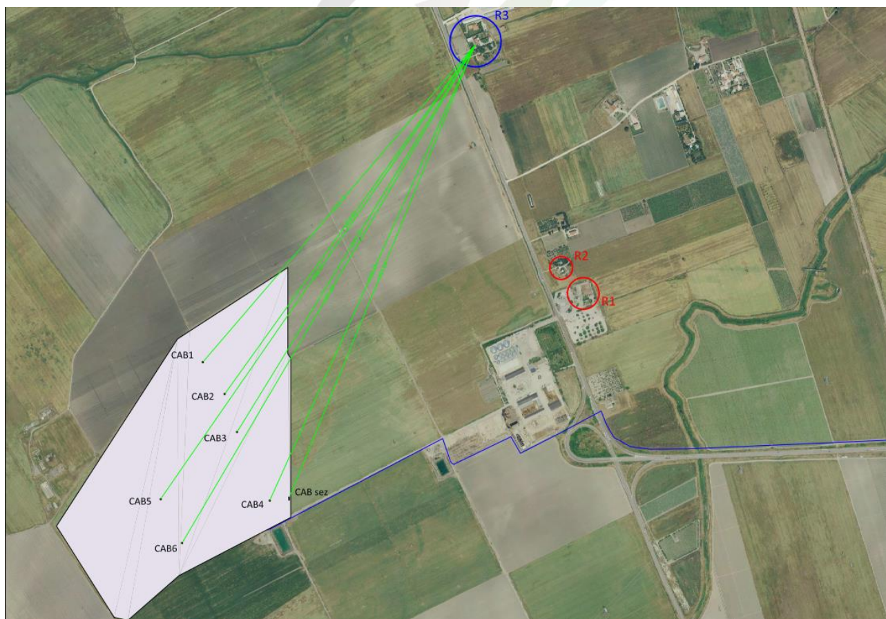
Figura 6-14: Distanza Cabine elettriche – Ricettore sensibile
