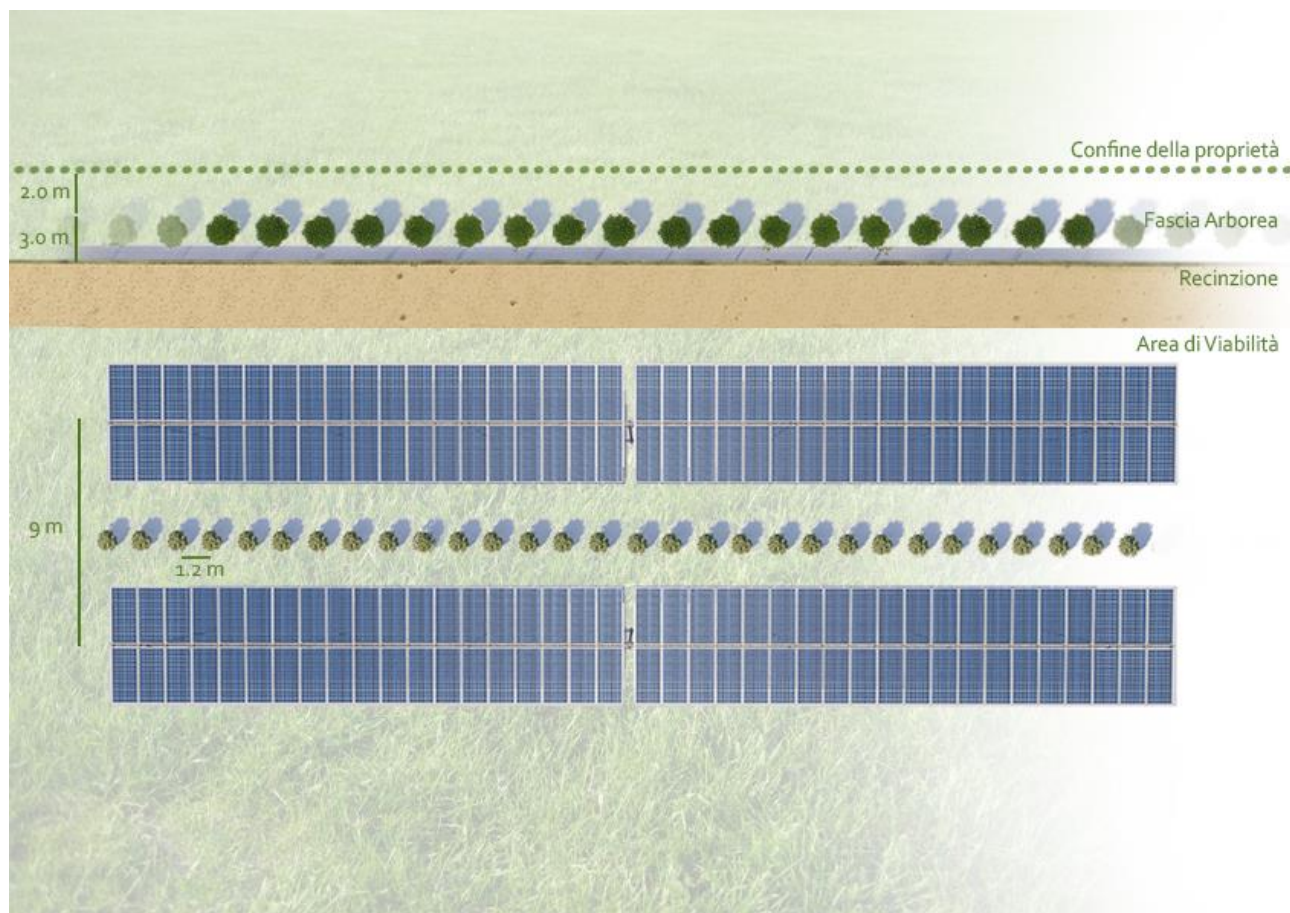
Figura 6-13: Schematizzazione dall'alto mandorleto – tracker – viabilità – recinzione – fascia arborea
