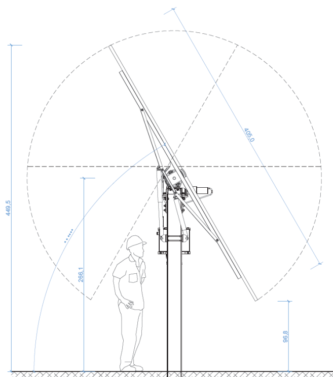
Figura 9. Sezione tipo del Tracker
