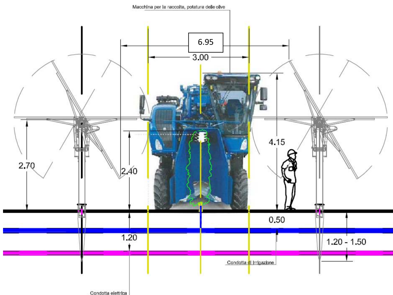
Figura 12. Sezione tipo impianto integrato
