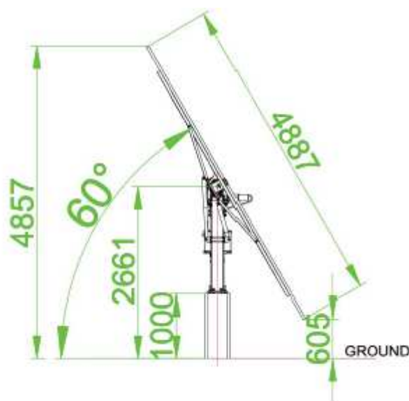
Fig. 9. Sezione tipo del Tracker
