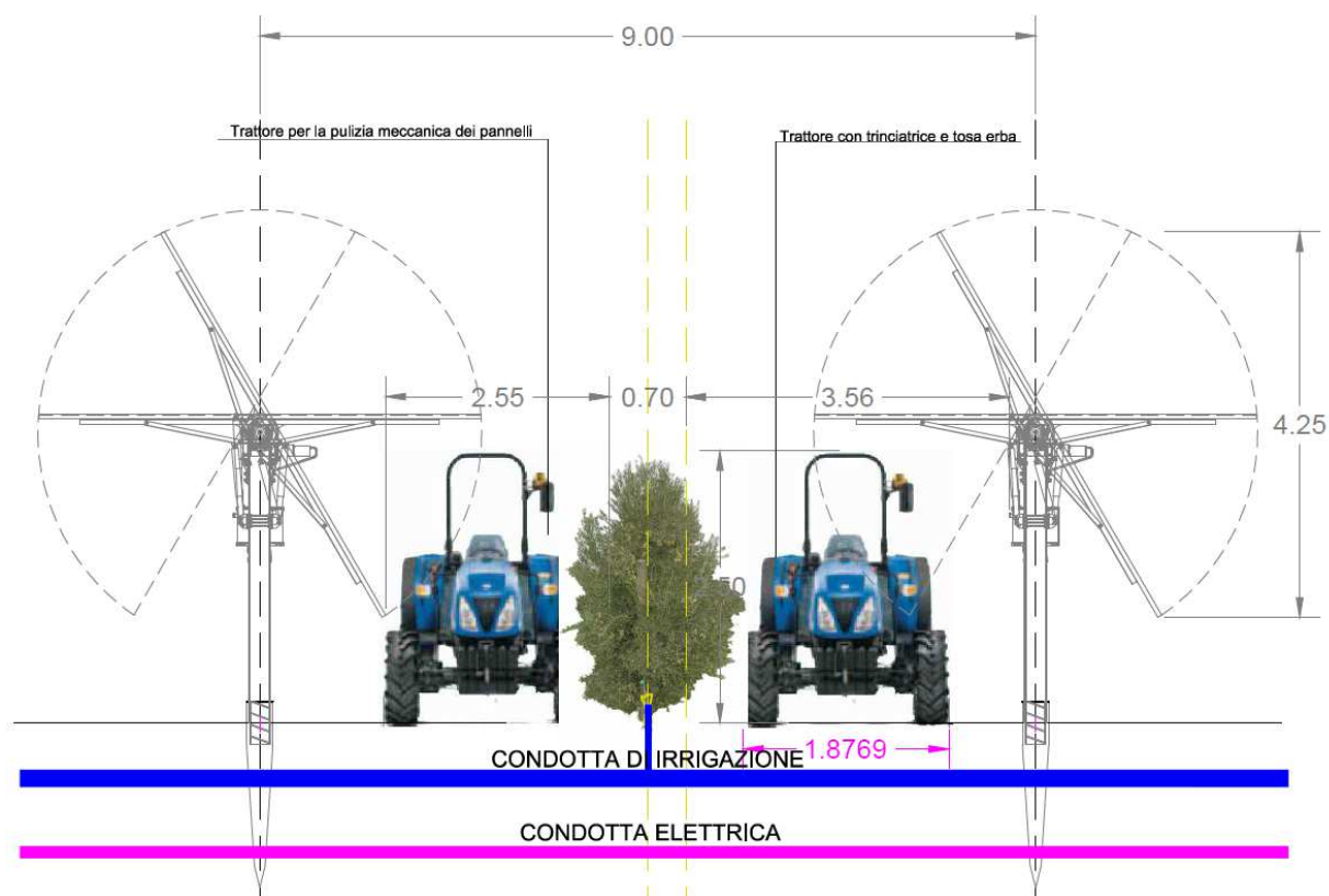
Fig. 14. Sezione tipo impianto integrato
