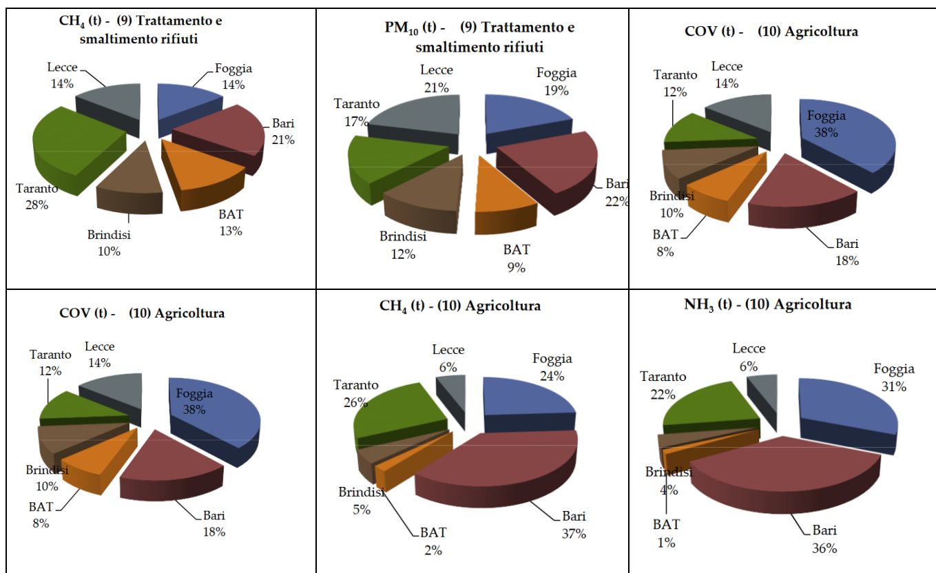
Fig. 22. Grafici delle emissioni in provincia di Foggia: per settori
