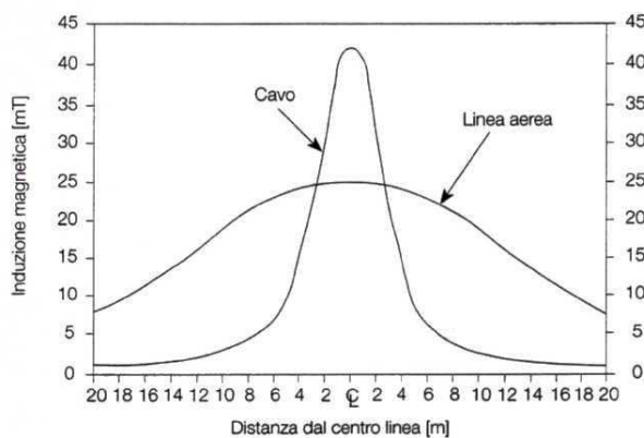
Fig. 28. Induzione magnetica per linea aerea e cavo interrato
