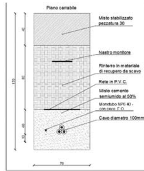
Figura 5-6 – Sezione tipo cavidotto su viabilità esistente non asfaltata
