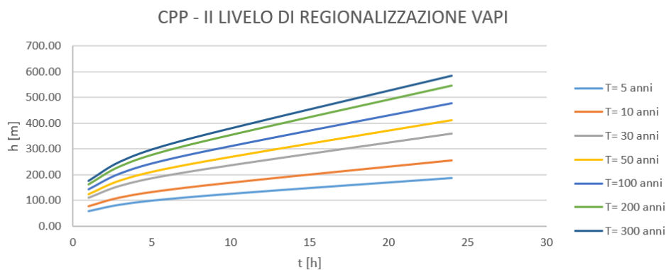
Figura 6-4- CPP ad assegnato tempo di ritorno
