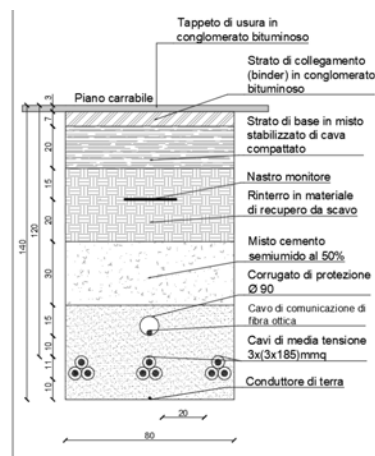
Figura 5-4- Sezione tipo cavidotto su viabilità esistente asfaltata
