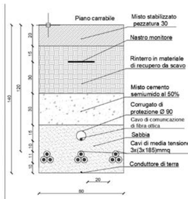
Figura 5-3 – Sezione tipo cavidotto su viabilità esistente non asfaltata
