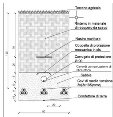
Figura 5-2- Sezione tipo cavidotto su terreno agricolo
