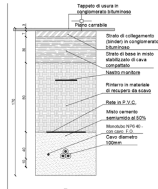
Figura 5-7- Sezione tipo cavidotto su viabilità esistente asfaltata
