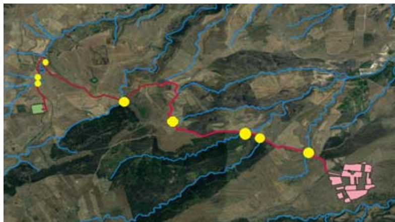
Figura 5-8- Punti di interferenza tra reticolo idrografico principale e cavidotto; in giallo i punti di interferenza;
