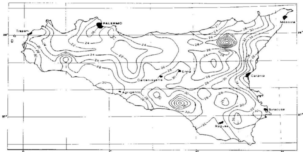
Figura 6-2 - Mappa isoparametrica del parametro n
