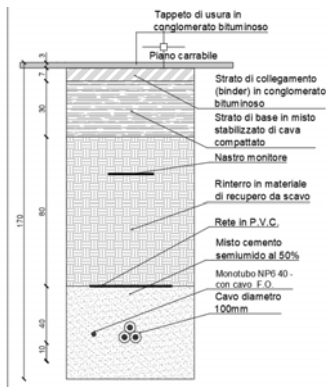
Figura 5-5- Sezione tipo cavidotto su terreno agricolo
