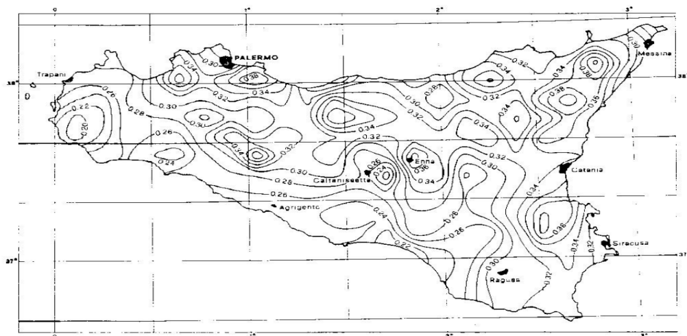
Figura 6-3- Mappa isoparametrica del parametro a
