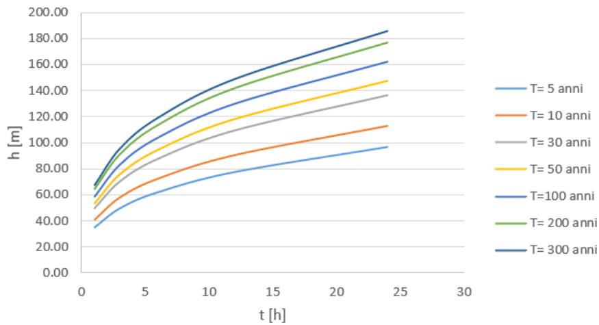
Figura 6-6 – Calcolo CPP con K_T di tabella 7
