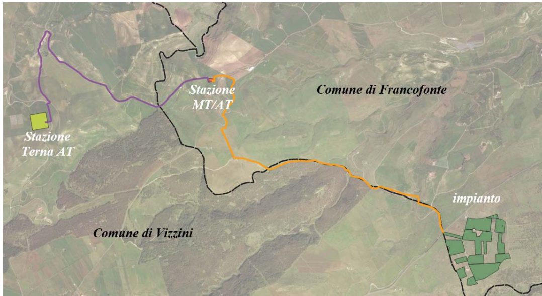
Figura 5-1- Tracciato del cavidotto
