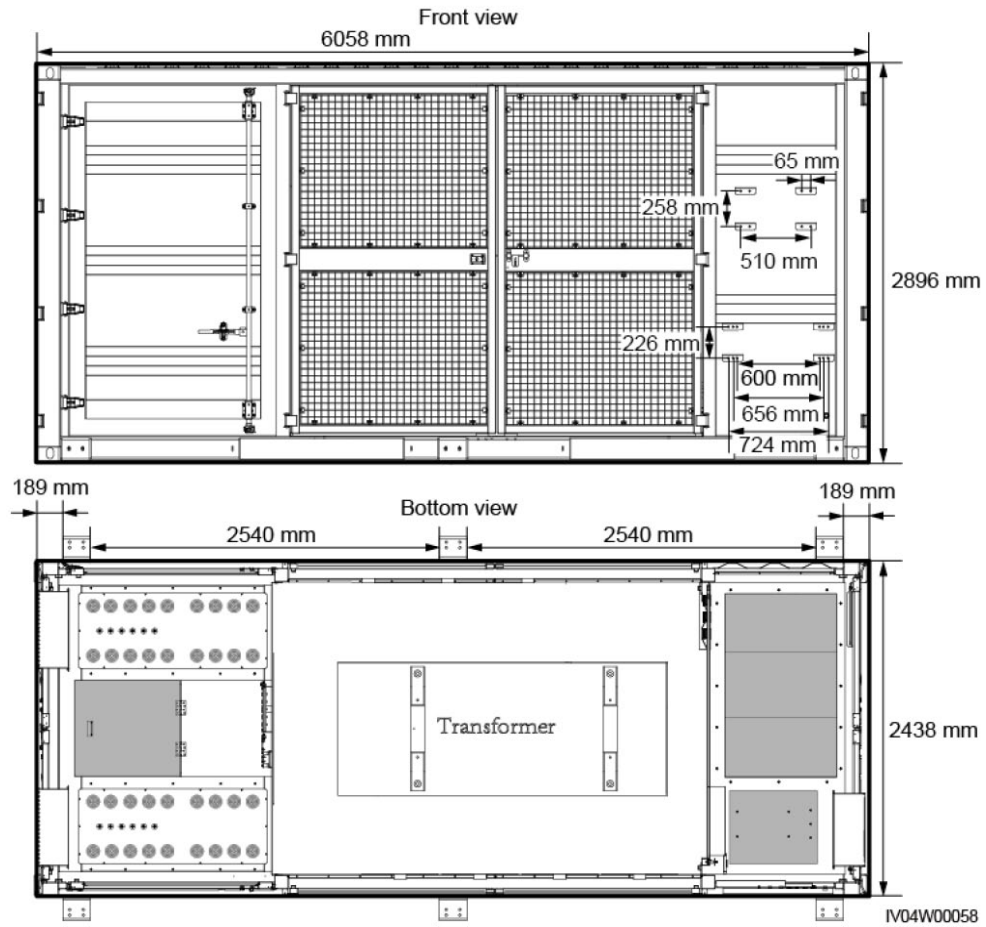
Figura 4 – dimensioni container
