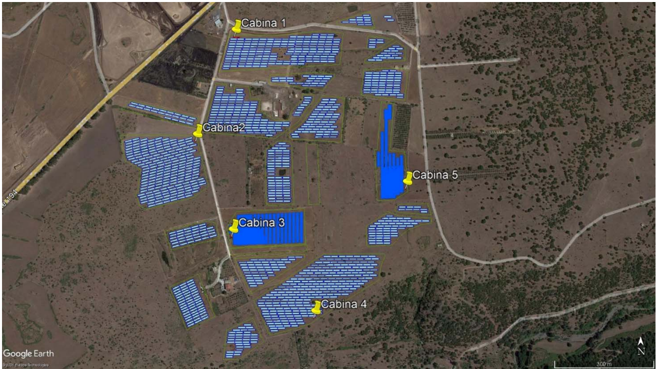
Figura 5 – Posizione cabine
