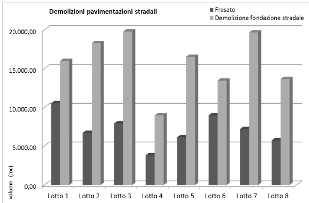
Figura E.3: Contributo di ogni lotto alla produzione di materiale di demolizione della sede stradale esistente
