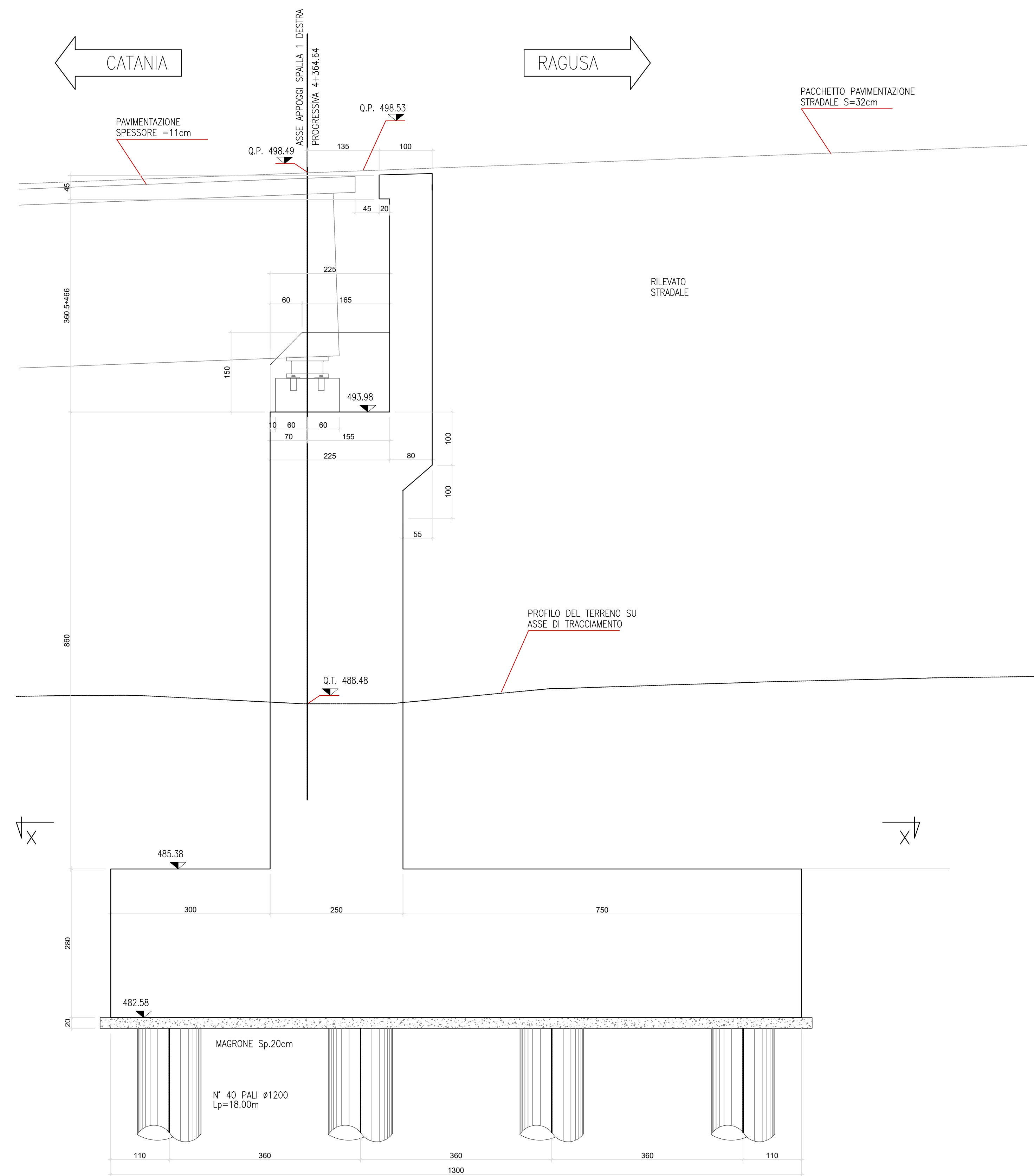
SPALLA Sp1Dx - (SEZIONE Y-Y)
