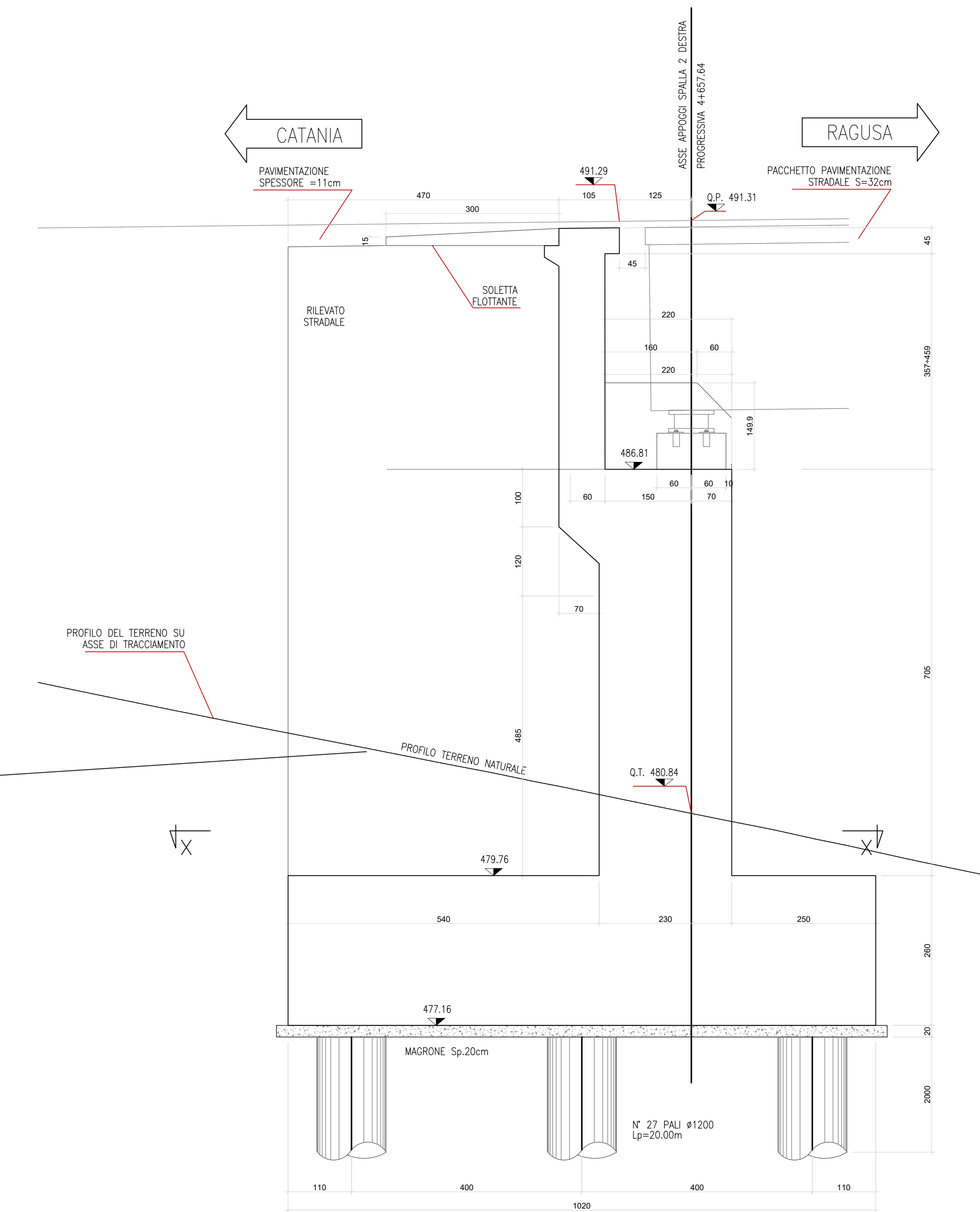
SPALLA Sp2Dx – (SEZIONE Z-Z)
