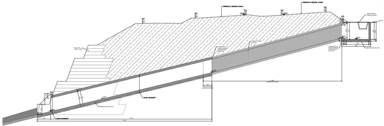
Figura 1-2 "Sezione con ricoprimento"
