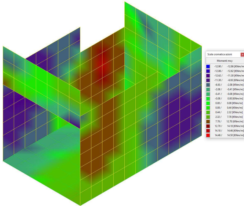
Figura 13-7 "Inviluppo momenti flettenti mxy"
