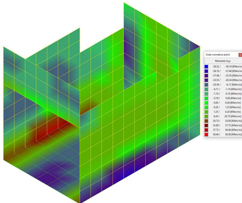
Figura 13-6"Inviluppo momenti flettenti myy"
