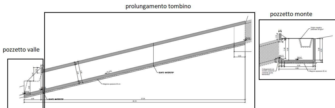
Figura 1-1 "Sezione"
