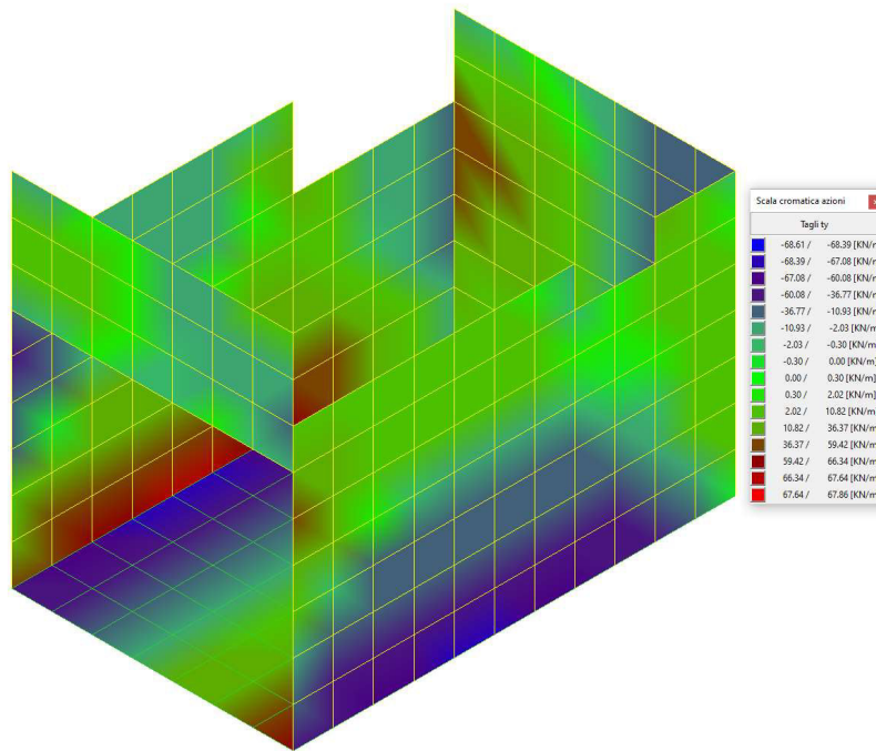
Figura 13-9 "Inviluppo tagli vy"
