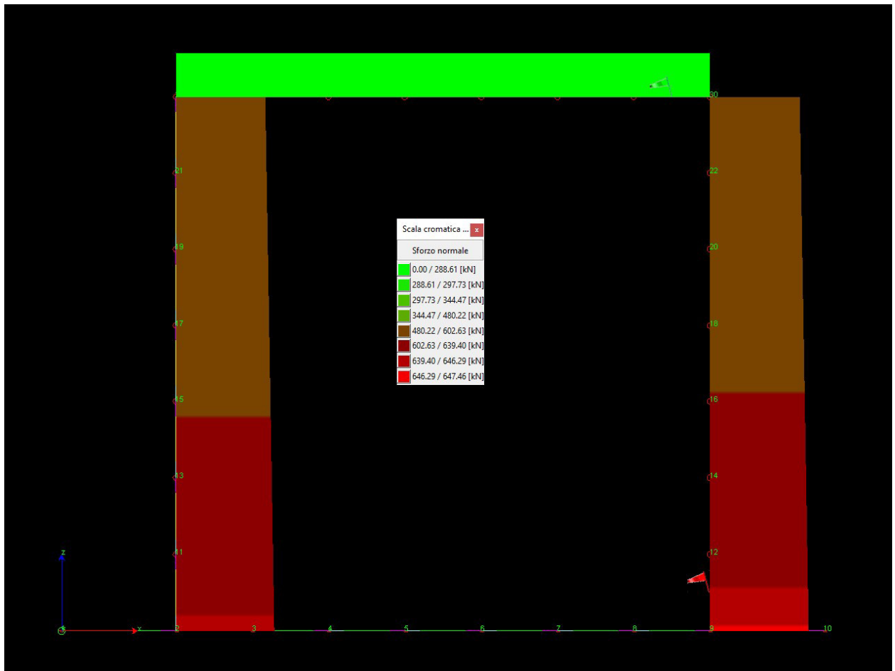
Figura 10-3 "Diagramma involuppo sforzo normale"
