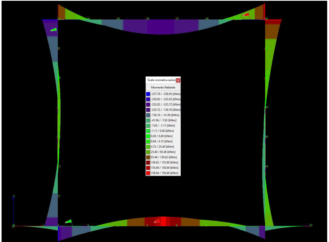
Figura 10-1 "Diagramma involuppo momenti flettenti"
