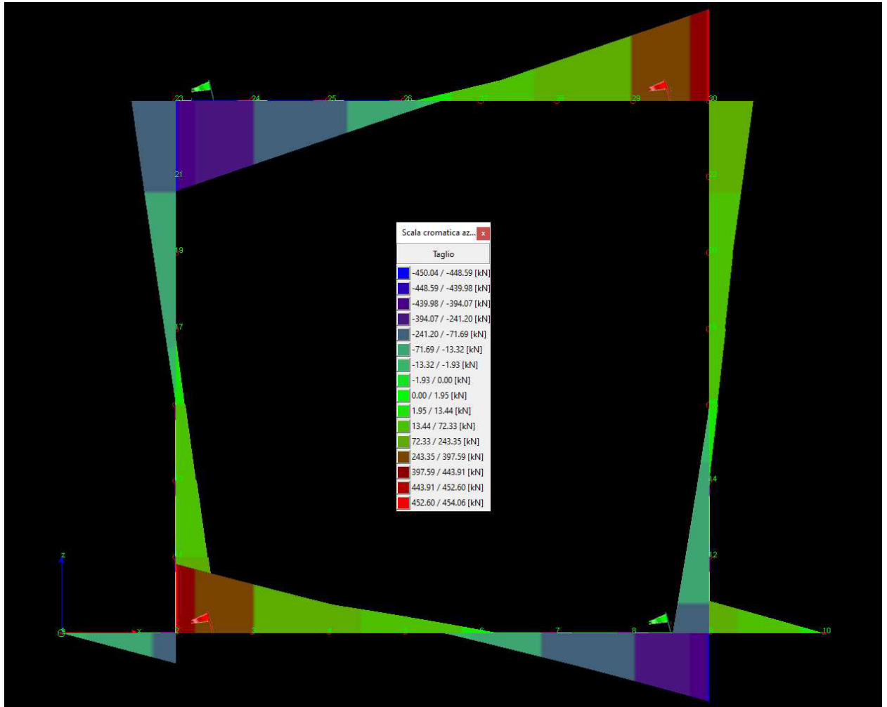
Figura 10-2 "Involucro diagramma taglio"
