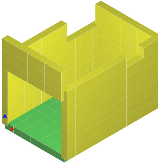
Figura 13-1 "Rappresentazione grafica del modello di calcolo"
