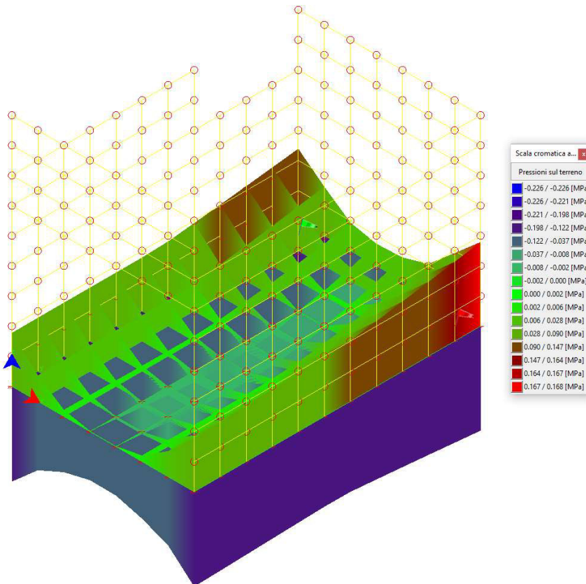
Figura 13-10 "Inviluppo pressioni terreno"
