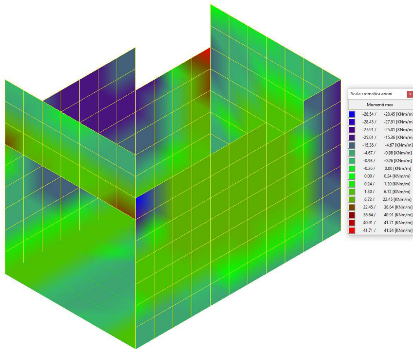
Figura 13-5"Inviluppo momenti flettenti mxx"
