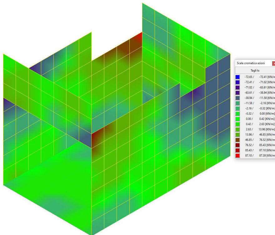
Figura 13-8 "Inviluppo tagli vx"
