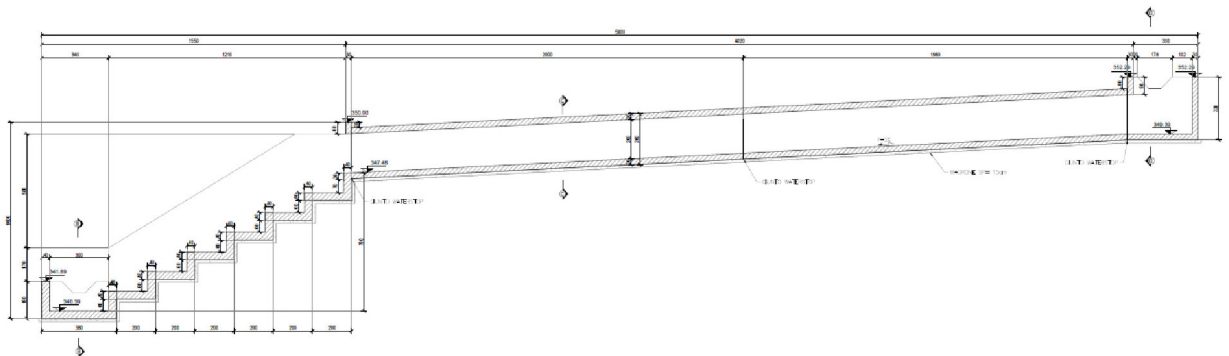
Figura 1-1 "Sezione longitudinale"
