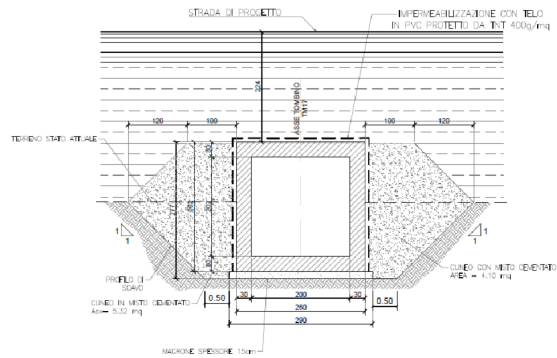
Figura 1-4 "Sezione trasversale"
