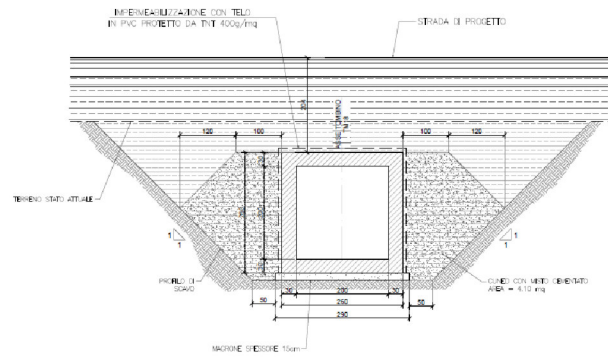
Figura 1-4 "Sezione trasversale"
