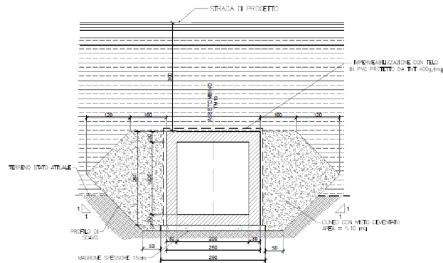
Figura 1-4 "Sezione trasversale"
