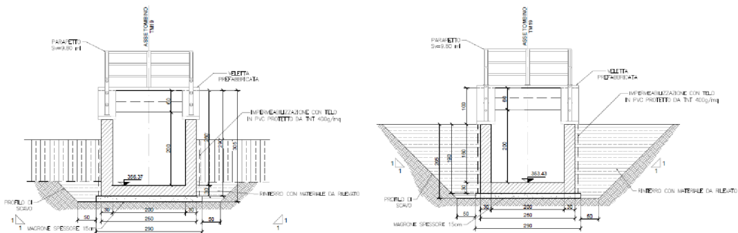
Figura 1- 5 "Sezione trasversale pozzetti di monte e di valle"
