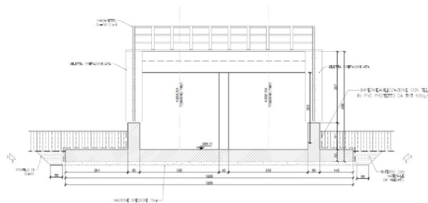
Figura 1-5 "Sezione trasversale pozzetti di monte"
