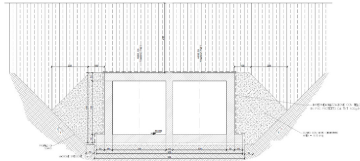
Figura 1-4 "Sezione trasversale"
