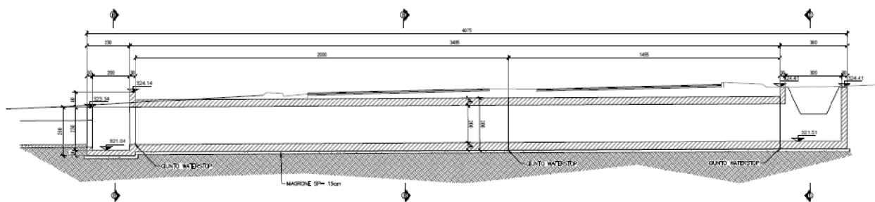
Figura 1-2 "Sezione longitudinale e rilevato stradale"
