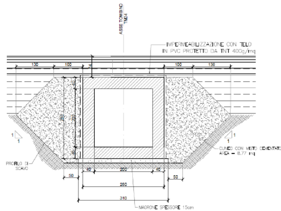
Figura 1-4 "Sezione trasversale"
