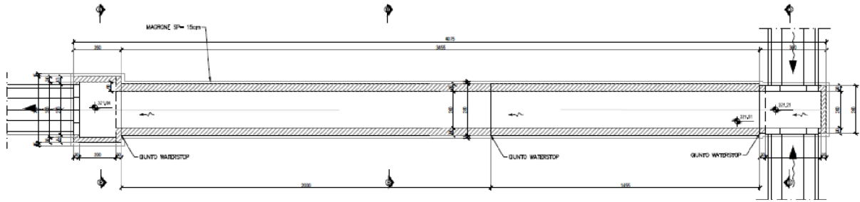
Figura 1-3 "Pianta"
