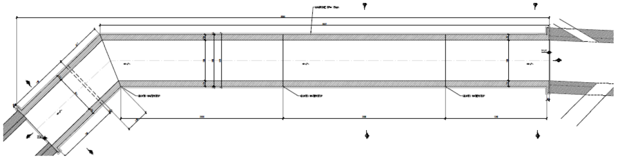
Figura 1-3 "Pianta"
