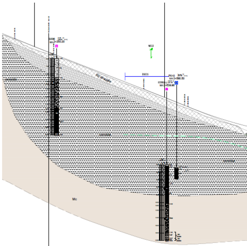
Figura 6.1: Stratigrafie di calcolo – Muro in T.R. OS51.
