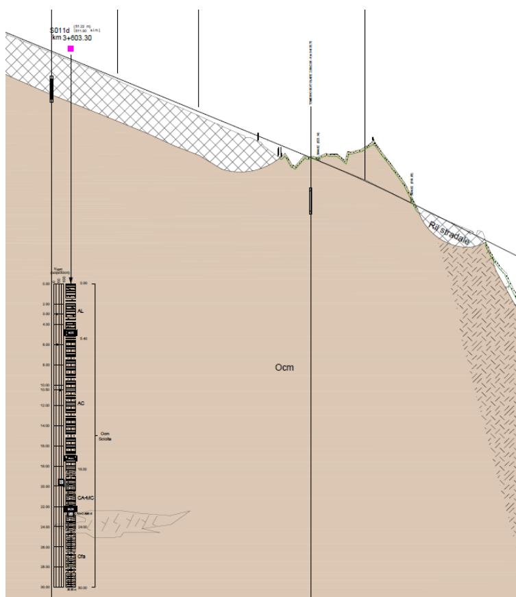
Figura 6.1: Stratigrafie di calcolo – Muro in T.R. OS53.
