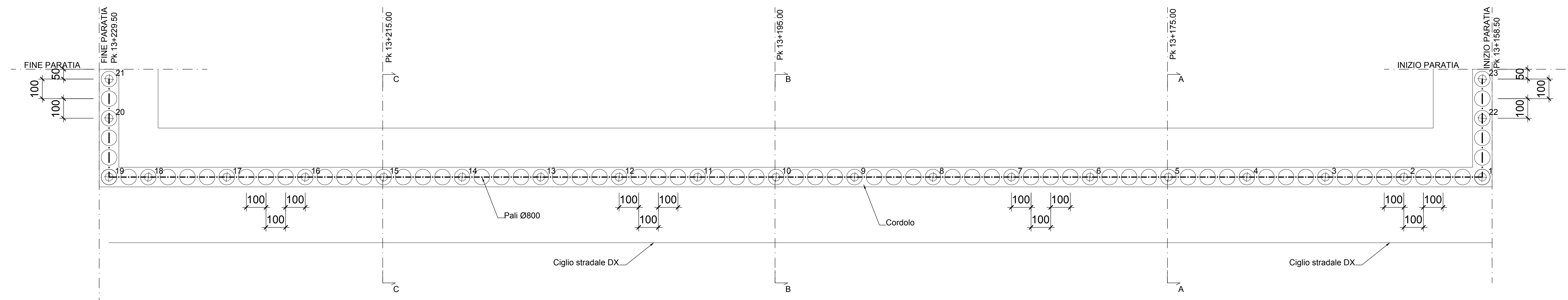
Prospetto Scala 1:100
