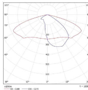
CURVA FOTOMETRICA
