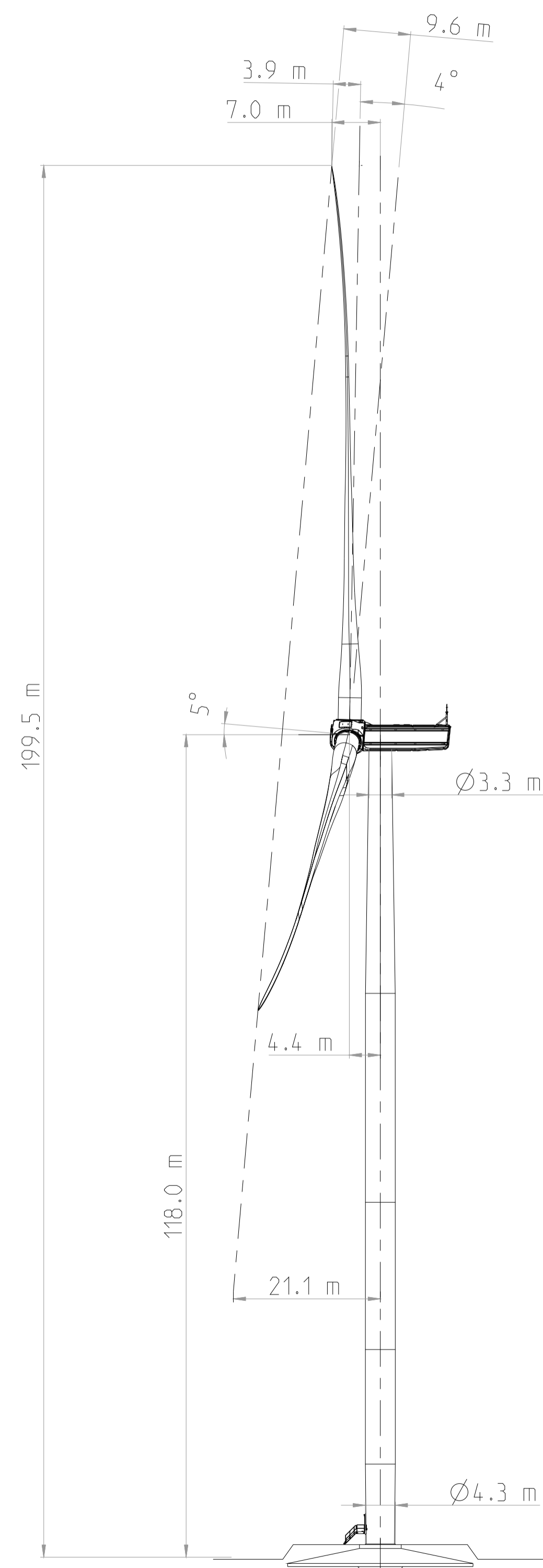
AEROGENERATORE TIPO DI PROGETTO - NORDEX 163
