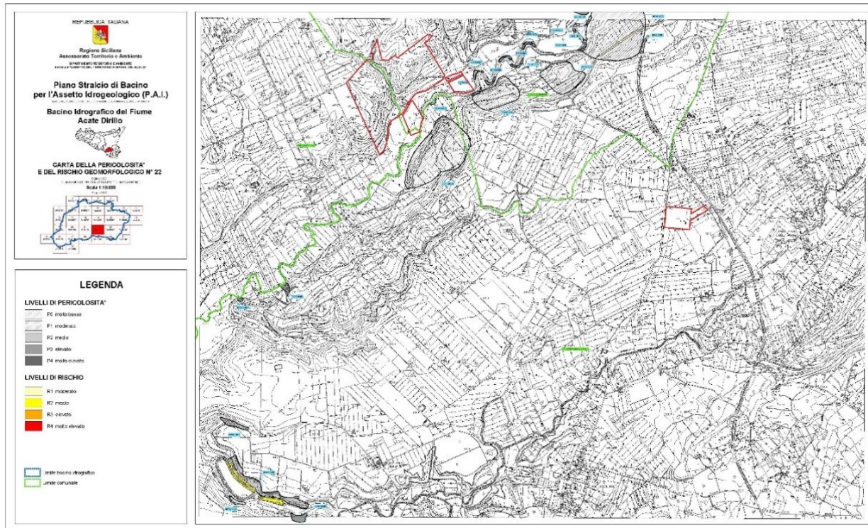
Figura 5 - Estratto fuori scale della "carta della Pericolosità e del Rischio Geomorfológico" allegata al Piano di Stralcio per l'Assetto Idrogeologico (P.A.I.)
