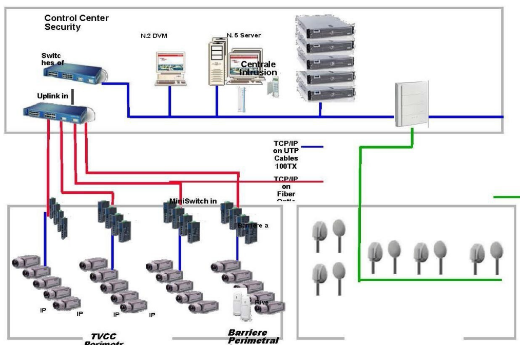
Figura 7 - Schema del Sistema di sorveglianza
