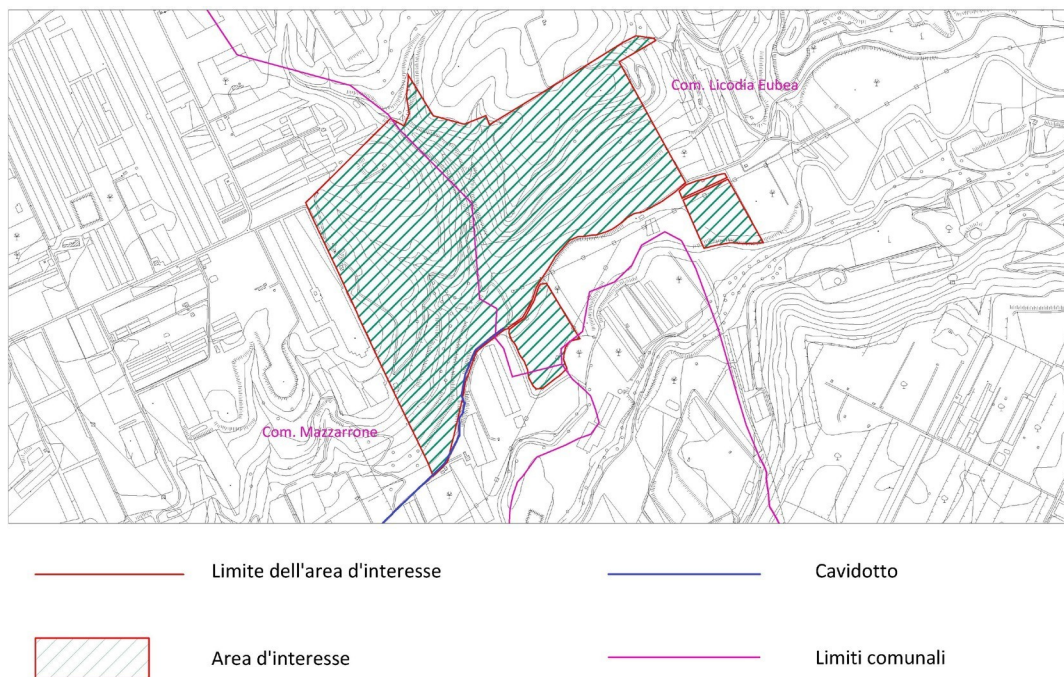
Figura 4 B - Inquadramento territoriale dell'area dell'impianto ricadente sul territorio di Mazzarrone (CT) e Licodia Eubea (CT) - località Leva, su C.T.R.
