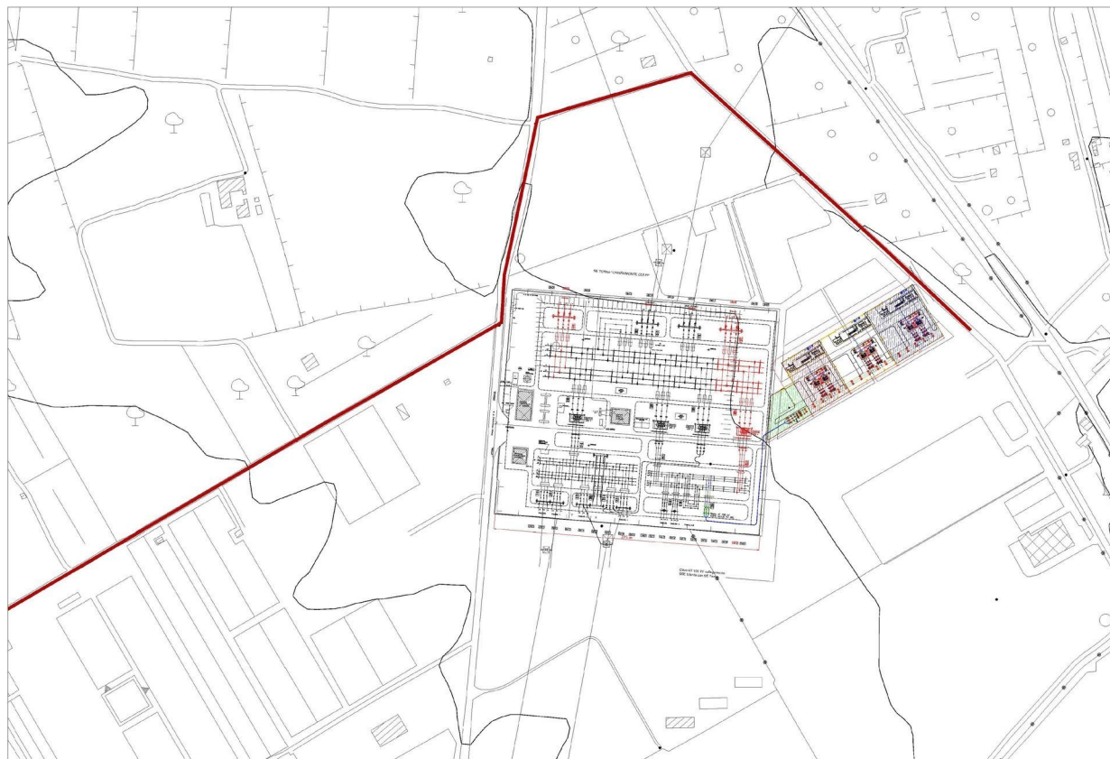
Figura 6 B - Layout dell'area della stazione ricadente sul territorio di Chiamonte Gulfi (RG) su C.T.R.
