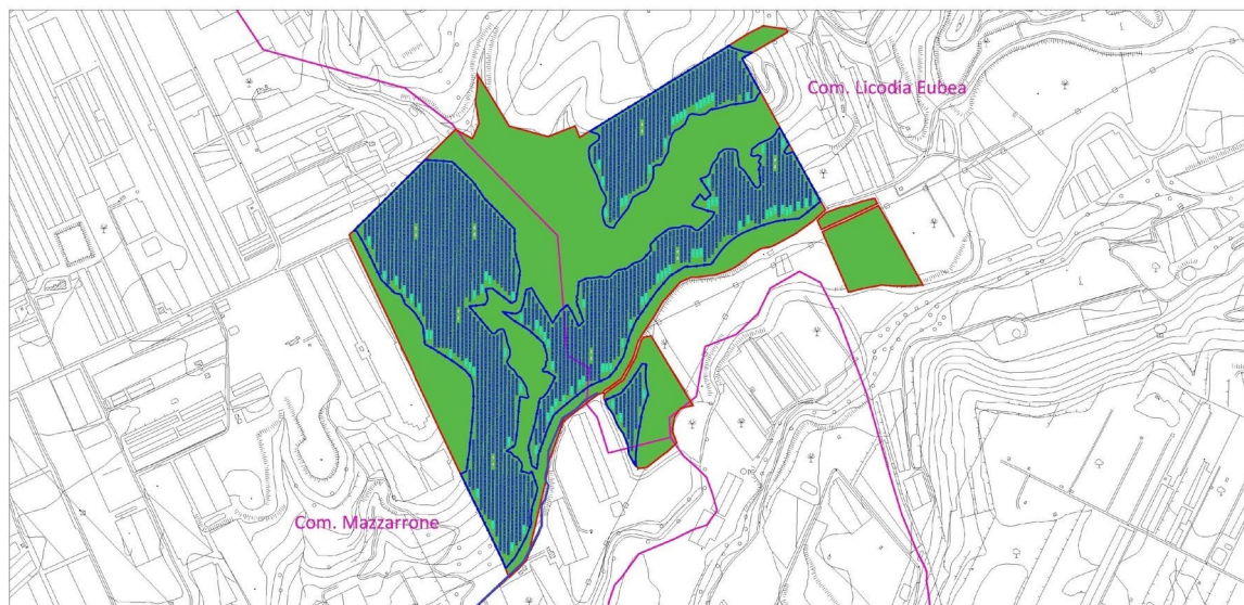
Figura 5 B - Inquadramento territoriale dell'area d'impianto ricadente sui territori di Licodia Eubea e Mazzarrone (CT) su catastale.
