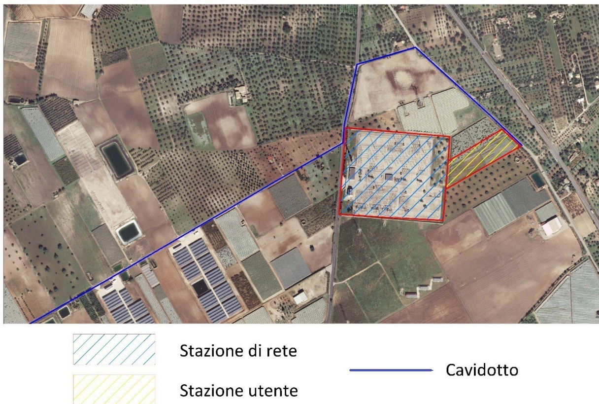
Figura 2 B - Ortofoto dell'area della stazione ricadente sul territorio di Chiaramonte Gulfi (RG)
