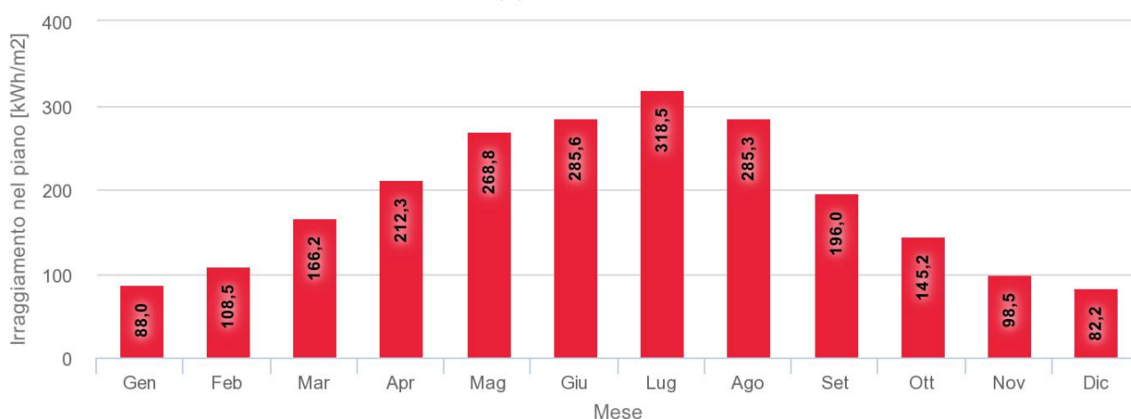
Figura 2 - Media mensile di irradiazione globale per metro quadro sul piano dei pannelli fotovoltaici.
