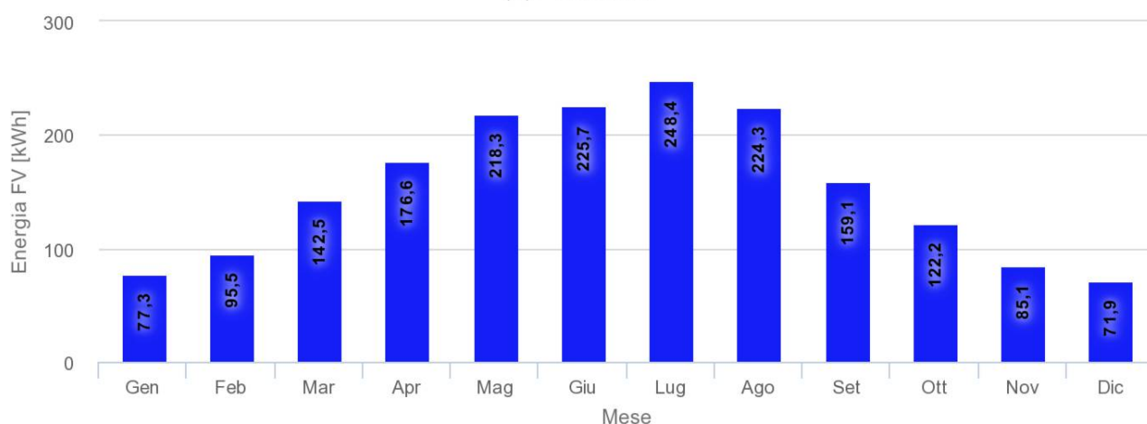
Figura 1 – Media mensile di produzione elettrica dell’impianto fotovoltaico.
