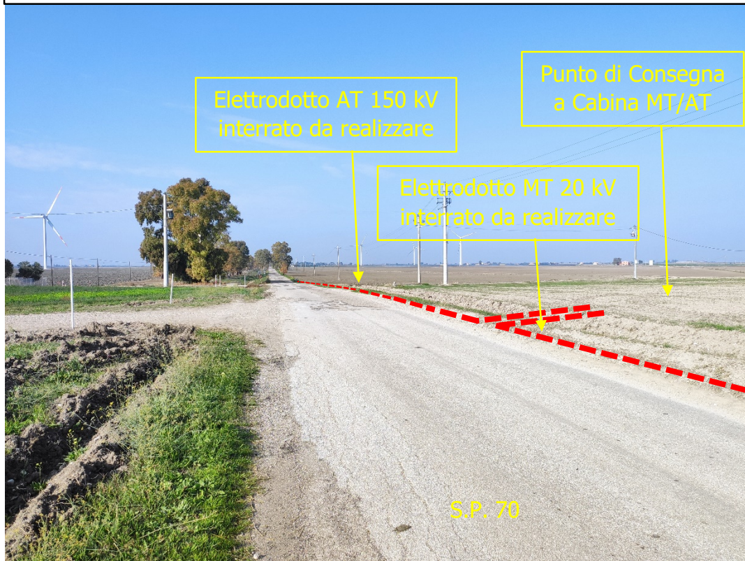
Foto n°8: Punto di Consegna a Cabina MT/AT
