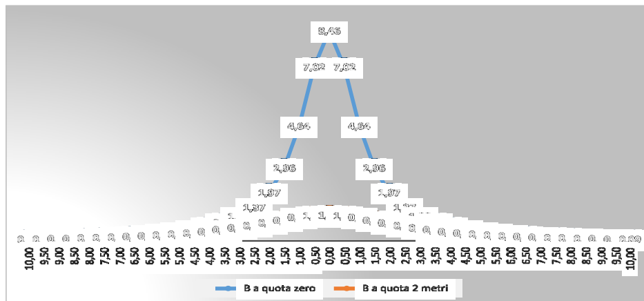
Fig. 1 Induzione Magnetica Cavo BT 600 mm 2
