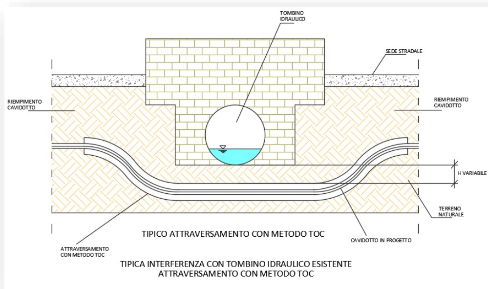
Figura 25- Schema tipico di risoluzione interferenza con tombino idraulico mediante l'utilizzo di metodo TOC
