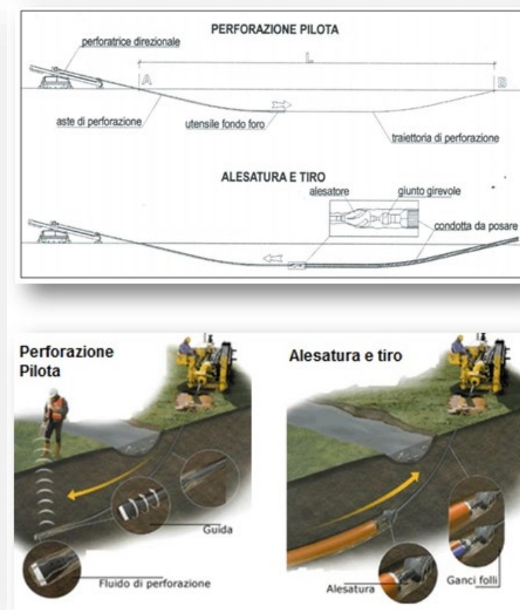
Figura 27 - Tecnologia di trivellazione orizzontale controllata (TOC)
