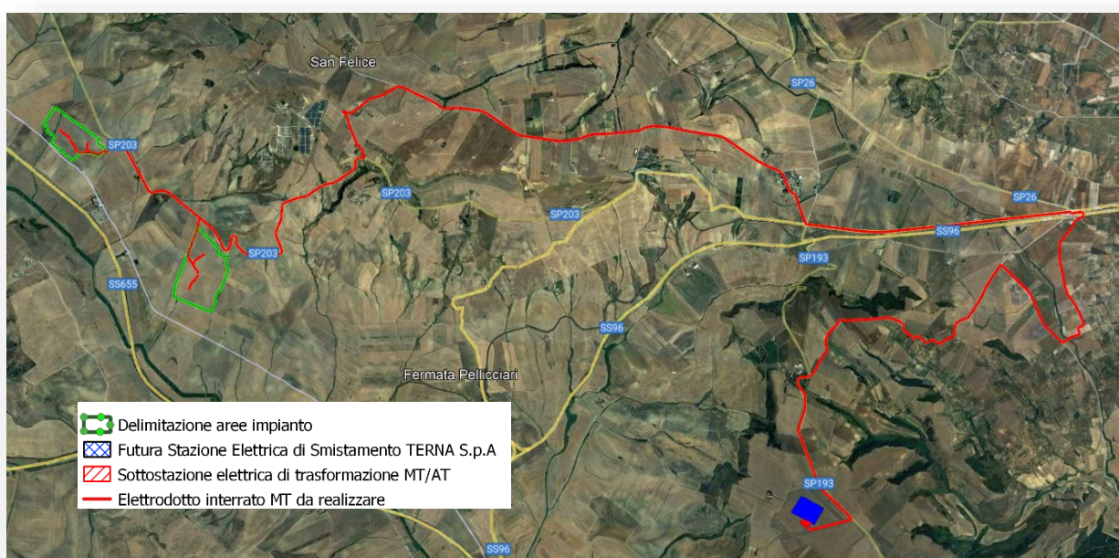
Figura 3 - Percorso dell'elettrodotto interrato MT da realizzare (tratto in rosso)
