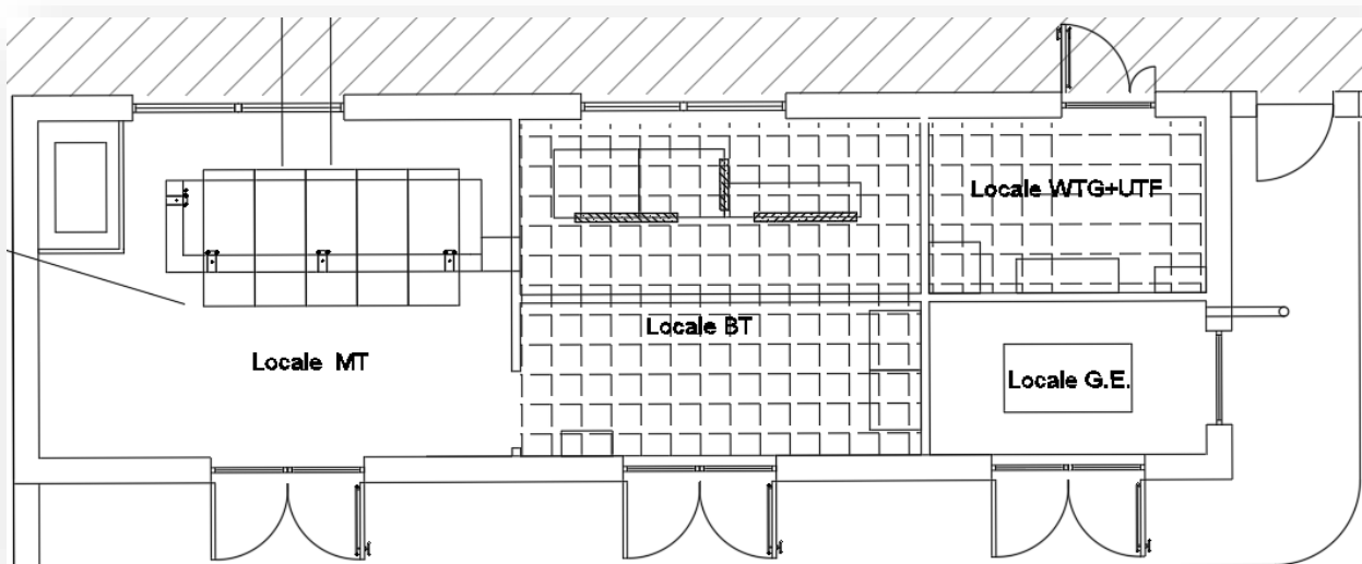
Figura 13- Estratto Elab. Q.12 Edificio di controllo SET
