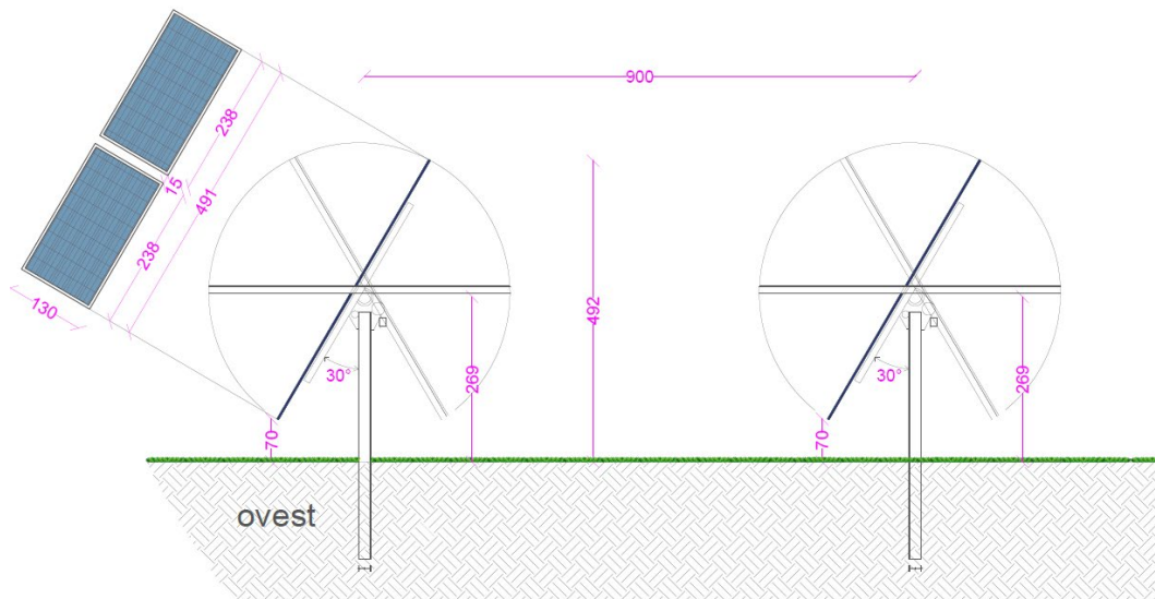
Figura 2 – Sezione tipo impianto nella configurazione tracker
