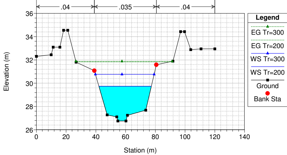
Da FCostanzo a FSanLeonardo Plan: stato_attuale
