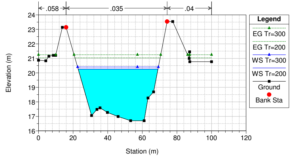
Da FCostanzo a FSanLeonardo Plan: stato_progetto
