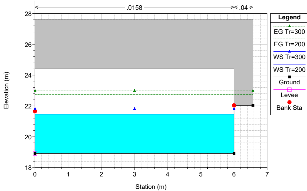
Da FCostanzo a FSanLeonardo Plan: stato_progetto
