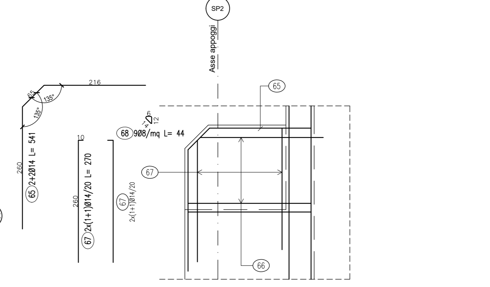
Spalla Sp2 Vista E-E Scala 1:50
