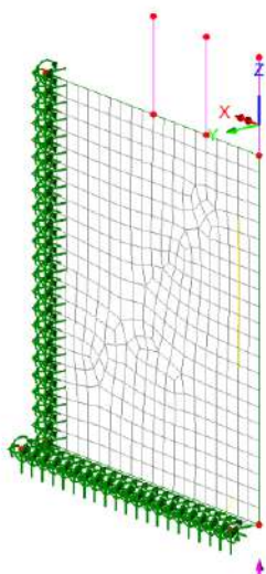
Figura 10.30 Muro ala - schema mesh E.F.
