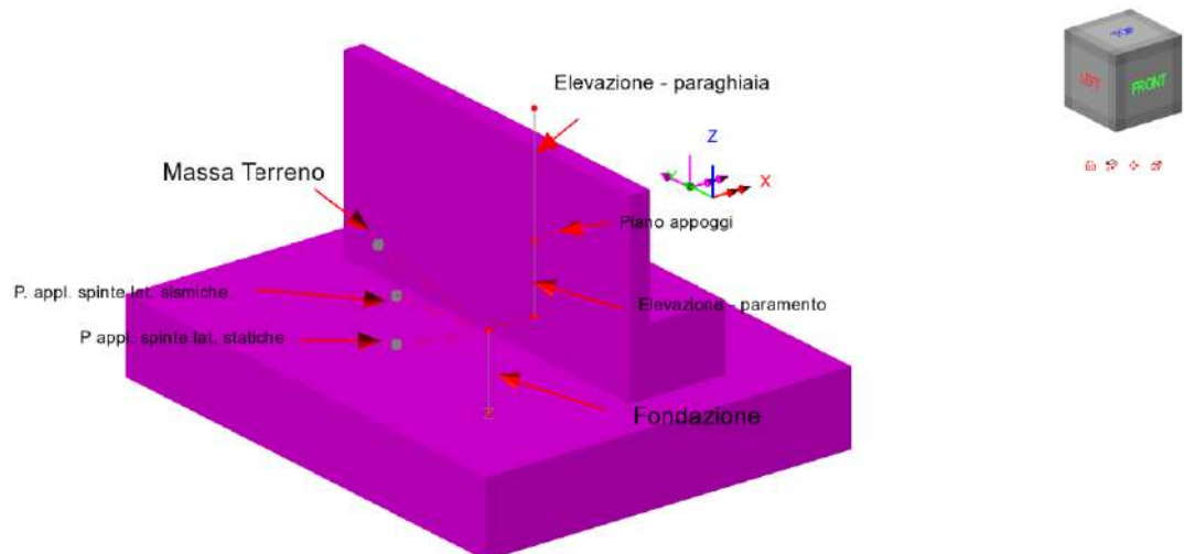
Figura 2.5 Modellazione spalla - layout E.F.
