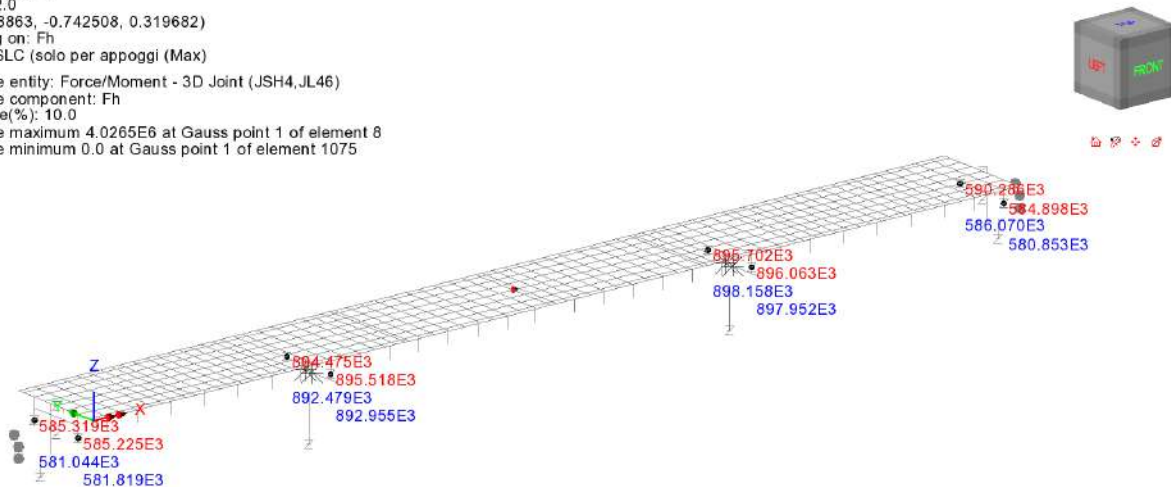
Figura 12.2 Reazioni orizzontali SLC - NomDP Analysis
