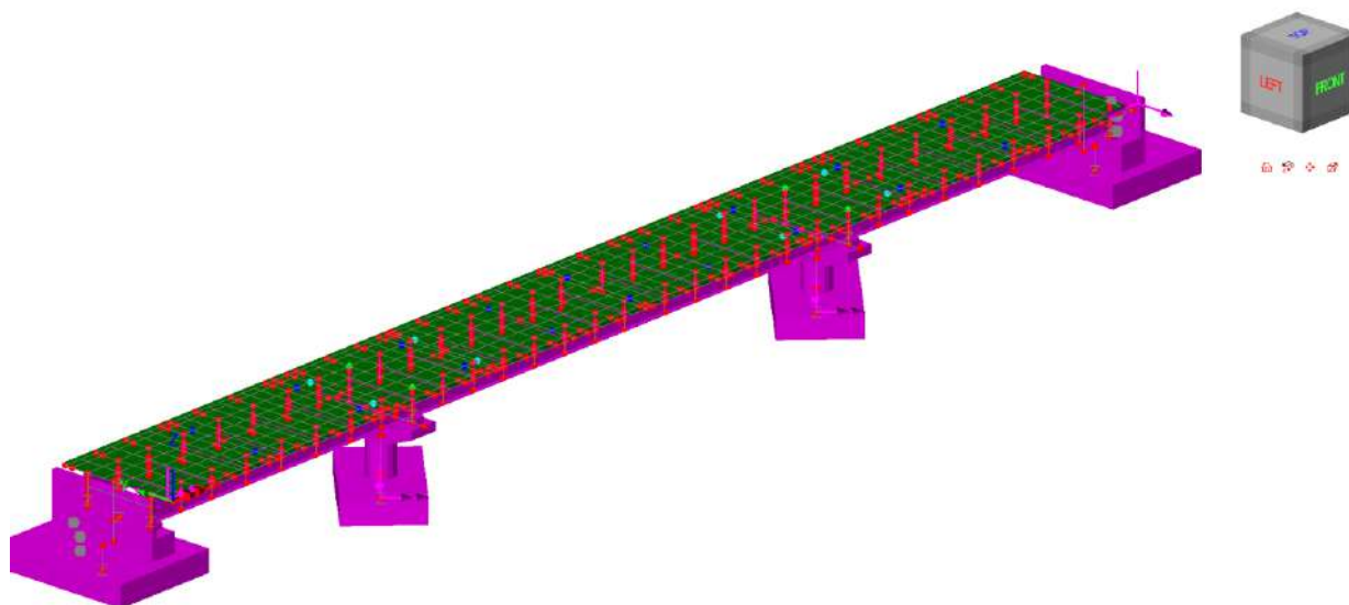
Figura 2.2 - Modello globale principale - Rendering
