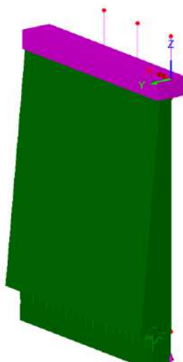
Figura 10.31 Muro ala - rendering modello E.F.
