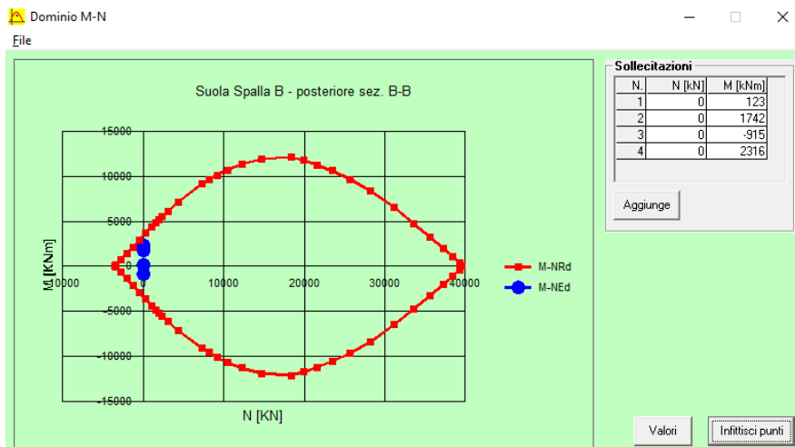
Figura 10.40 Dominio di resistenza sezione B-B
