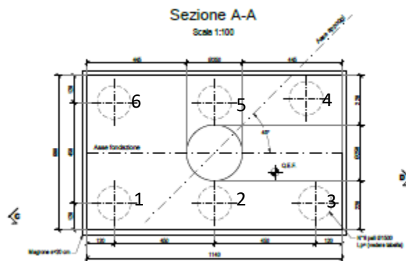
Figura 10.25: Pianta del plinto con numerazione pali
