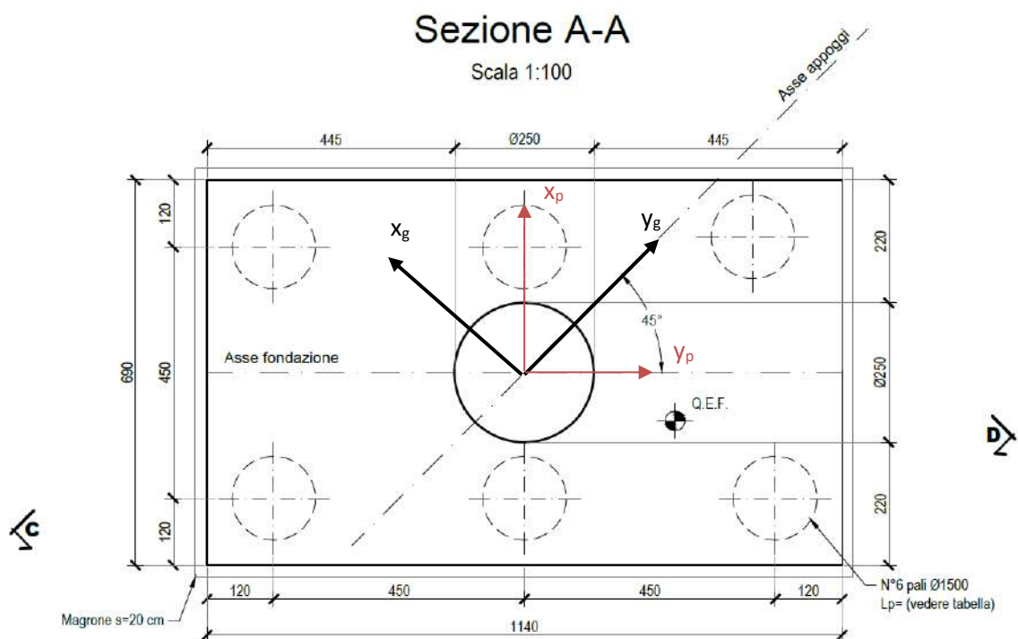
Figura 9.1 : Pianta fondazione pila
