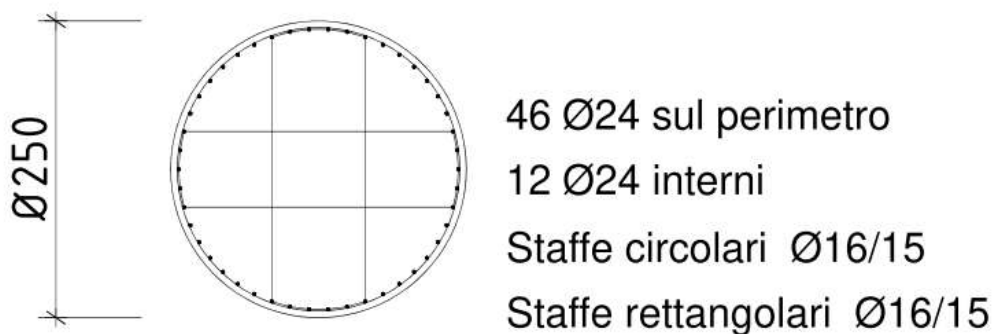
Figura 10.1: Dimensioni ed armatura pila 1
