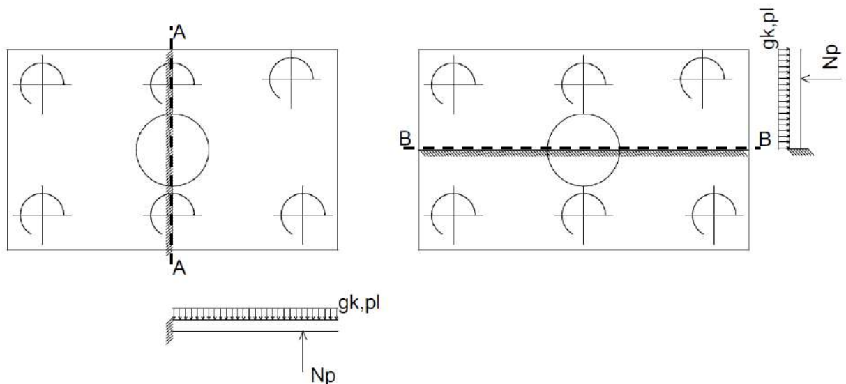
Figura 10.26: Schemi di calcolo per statica trasversale e longitudinale
