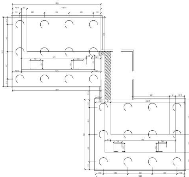
Figura 1.8 Disallineamento spalle via dx/sx
