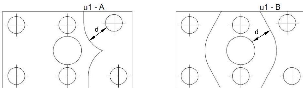
Figura 10.27 Perimetri di controllo per verifica a punzonamento
