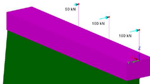
Figura 10.32 Muro ala - dettaglio modellazione urto
