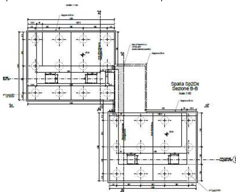
Figura 9.2 Schema fondazioni spalla
