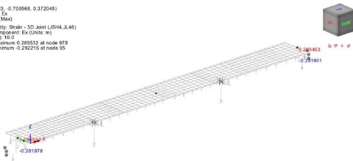
Figura 12.11 Escursione lg giunti SLV – NomDP analysis
