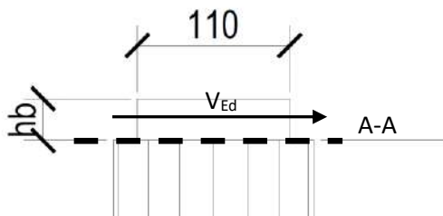
Figura 10.19 Sezione di verifica meccanismo "shear friction "
