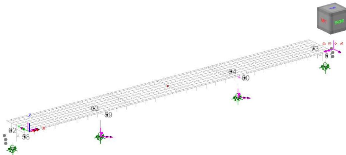
Figura 2.7: Vincoli esterni e numerazione degli elementi di molla concentrata presenti nel modello
