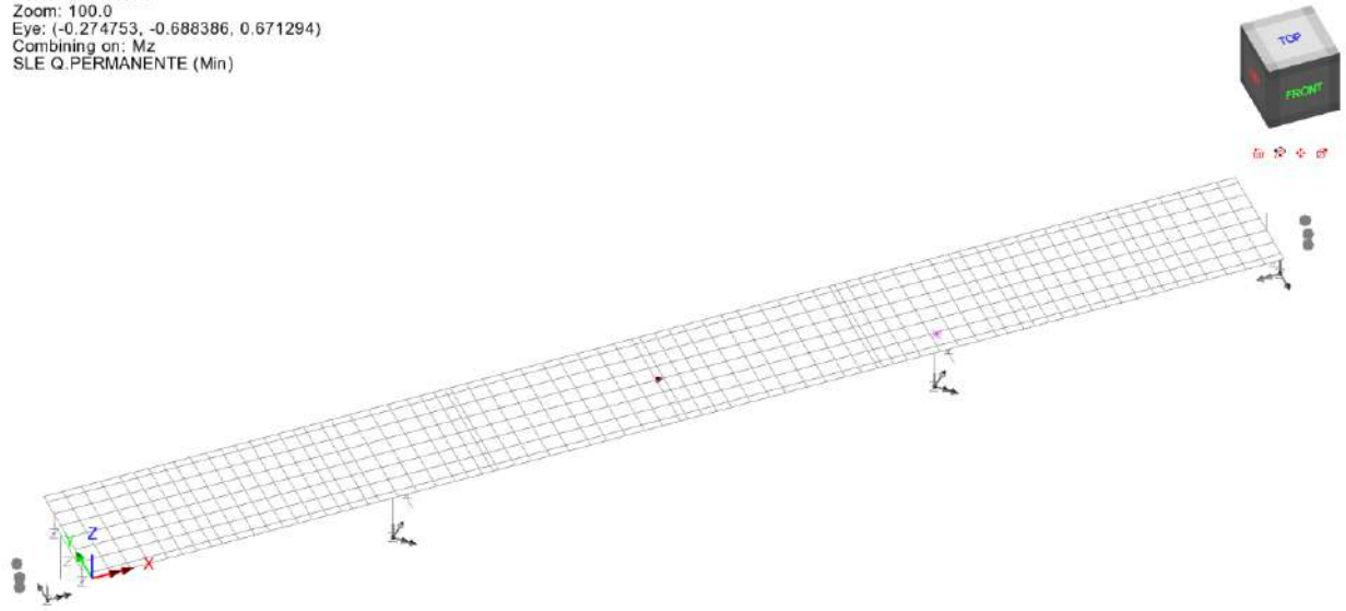
Figura 8.5 Sistema riferimento sollecitazioni in fondazione
