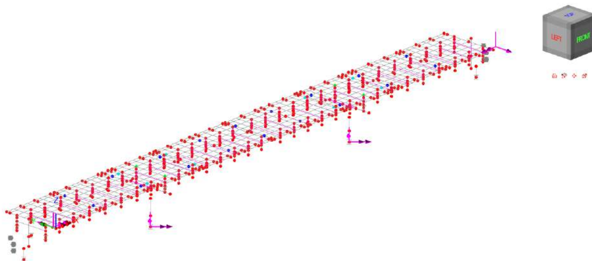
Figura 2.1 - Modello globale principale – layout E.F.
