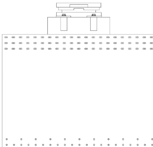
Figura 10.8 schema armatura a flessione pulvino
