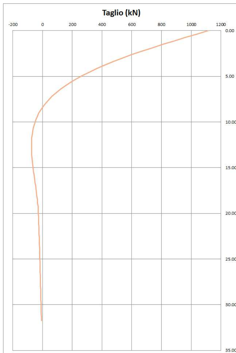
Figura 10.43 Diagramma di flessione e taglio massimi sul palo delle spalle 1 e 2
