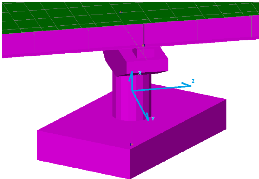
Figura 10.3: Sistema di riferimento elementi pila 1
