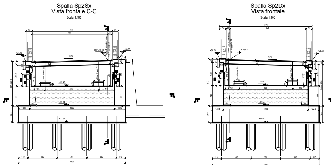
Figura 1.7: Vista frontale spalle SP2
