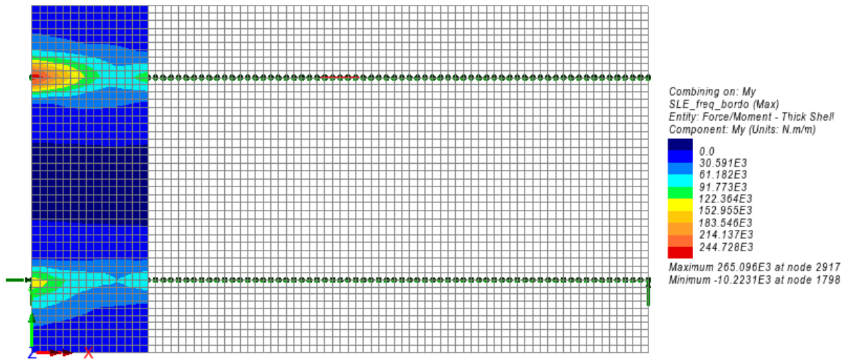
Figura 10.29: SLE frequente – Momento My (max)
