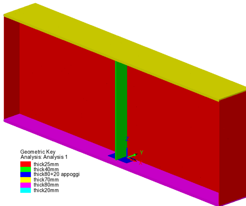
Figura 11.6 Rendering + spessori di calcolo – lato interno
