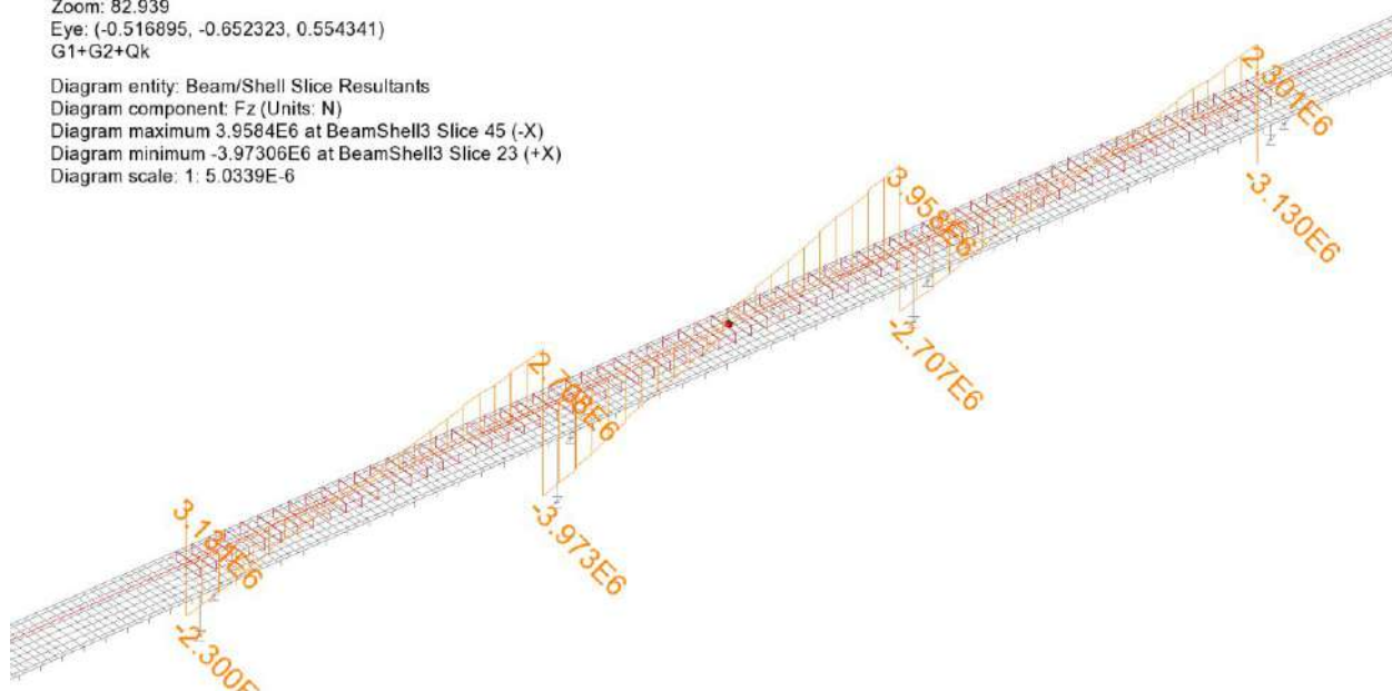
Figura 12.6 Fz - G1+G2+Q - modello F.E.M. originale
