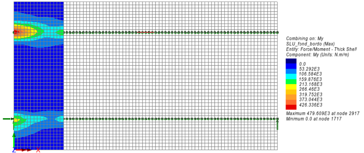
Figura 10.23: SLU fondamentale – Momento My (max)
