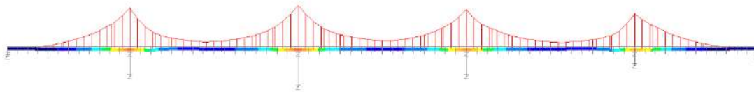
SLU fondamentale My max
