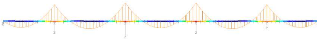
Gk1 - Peso proprio soletta - My
