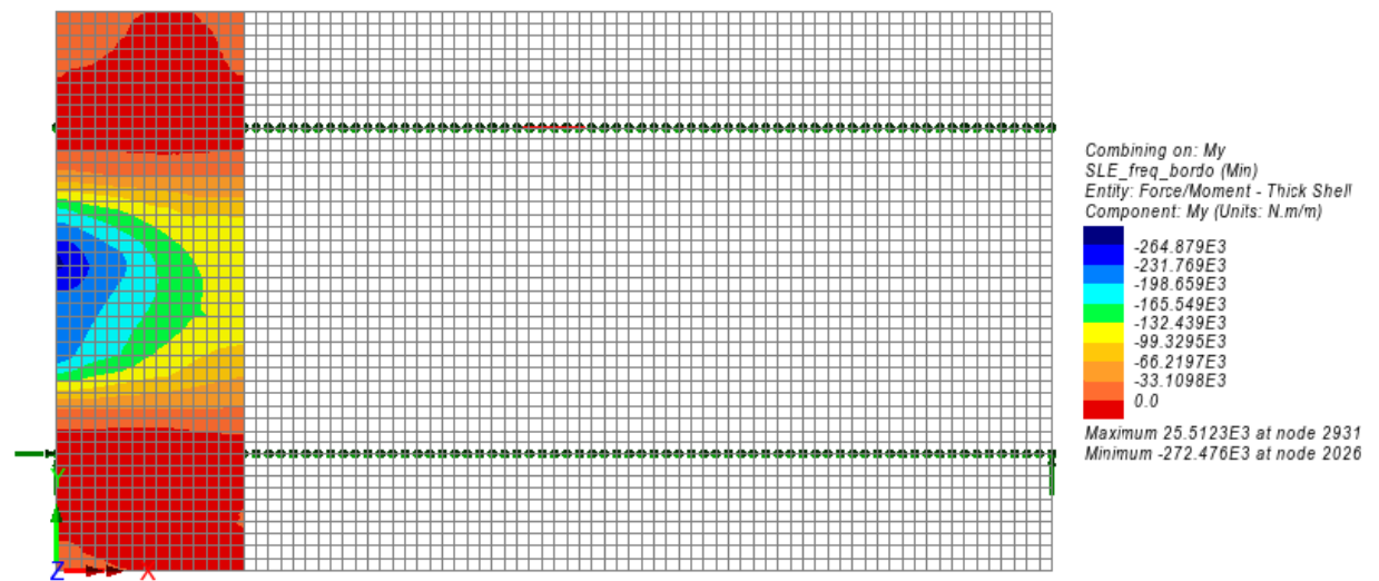
Figura 10.30: SLE frequente – Momento My (min)
