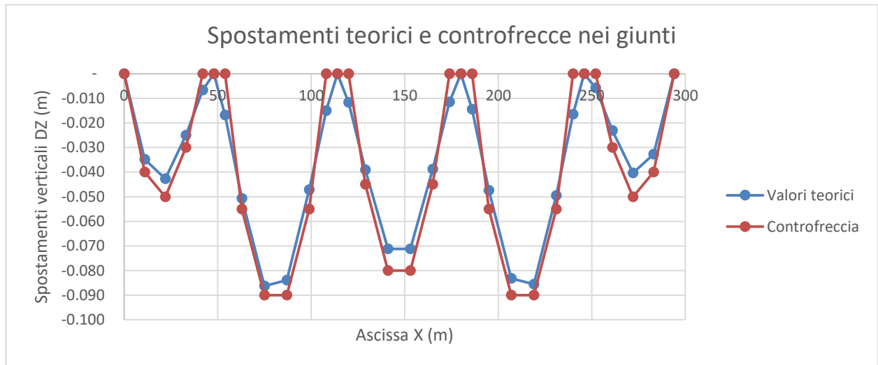
Figura 6.4: Freccie teoriche e controfreccie dovute a peso proprio, permanente ed aliquota di traffico
