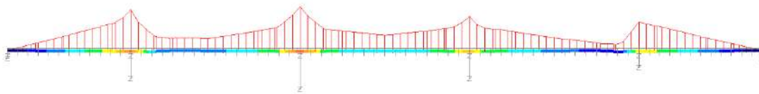
Qk - Traffico caratteristico My max
