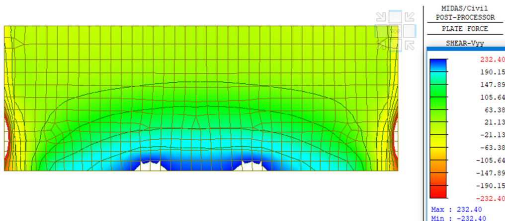
Figura 31 – Sollecitazioni taglianti limitate al valore di taglio resistente in presenza di specifica armatura resistente (paraghiaia)
