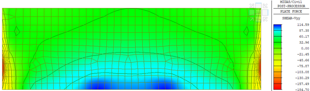
Figura 16 – Taglio Vyy (involuppo)
