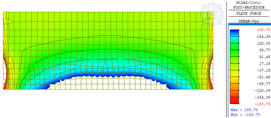
Figura 29 – Sollecitazioni taglianti limitate al valore di taglio resistente in assenza di specifica armatura resistente (paraghaia)
