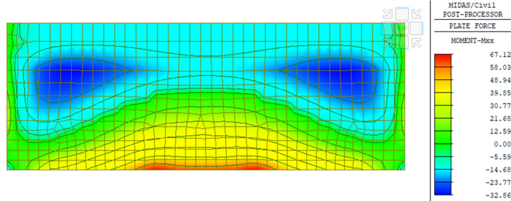
Figura 9 – Momento flettente Mxx (involuppo)
