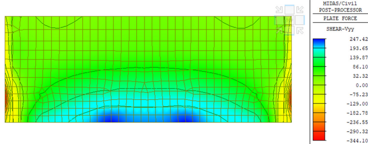
Figura 12 – Taglio Vyy (involuppo)
