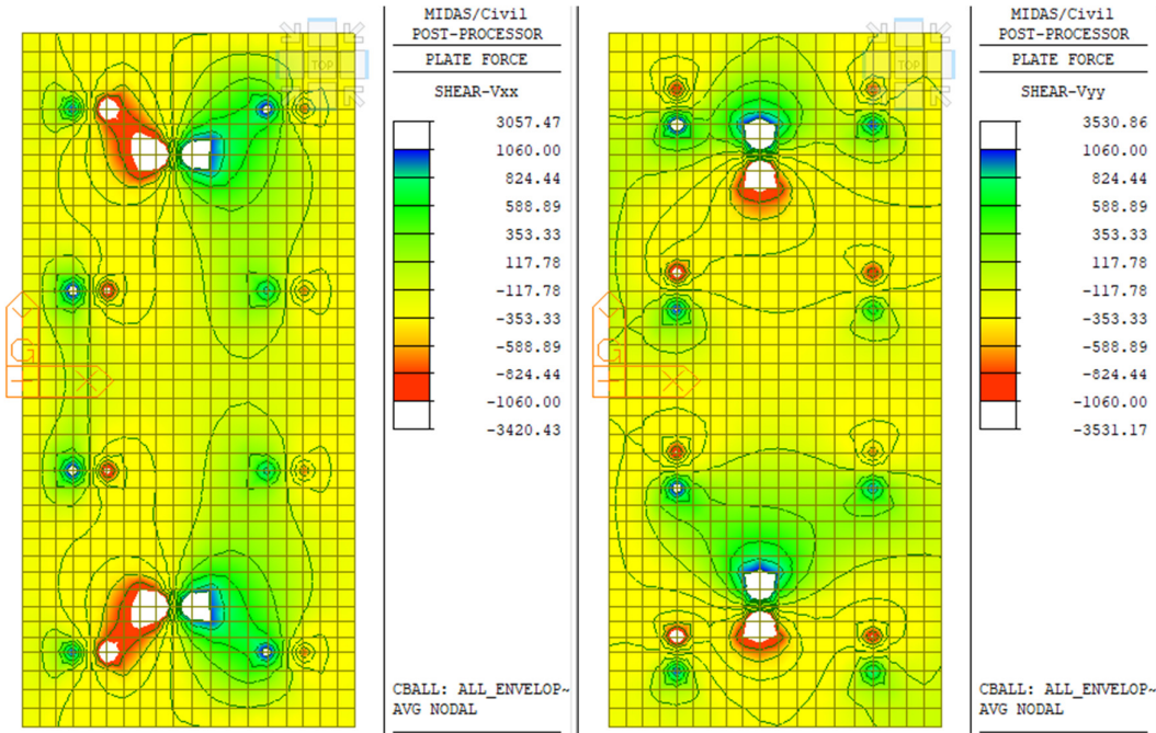
Figura 32 – Sollecitazioni taglianti limitate al valore di taglio resistente in presenza di specifica armatura resistente (fondazione)
