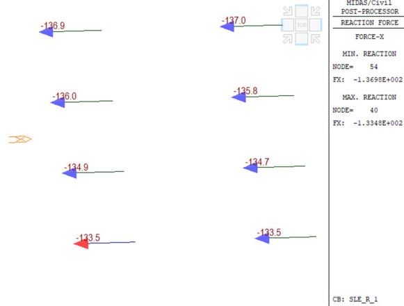
Figura 24 – Reazioni in direzione longitudinale
