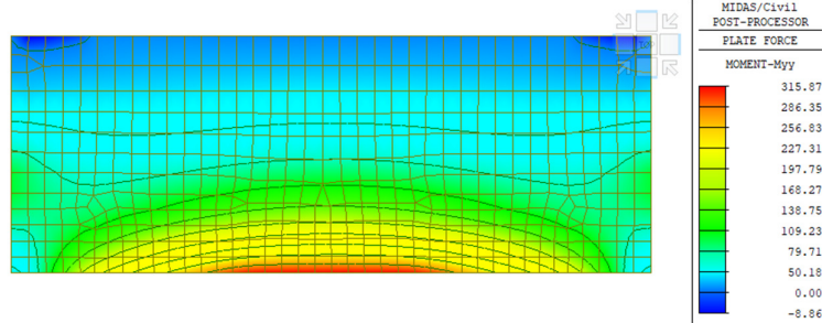
Figura 10 – Momento flettente Myy (involuppo)
