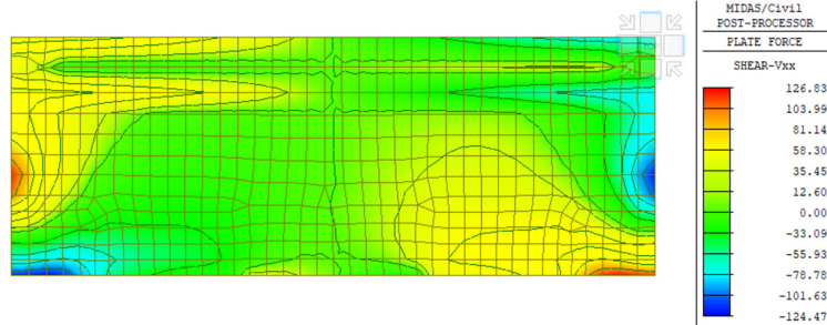
Figura 11 – Taglio Vxx (involuppo)
