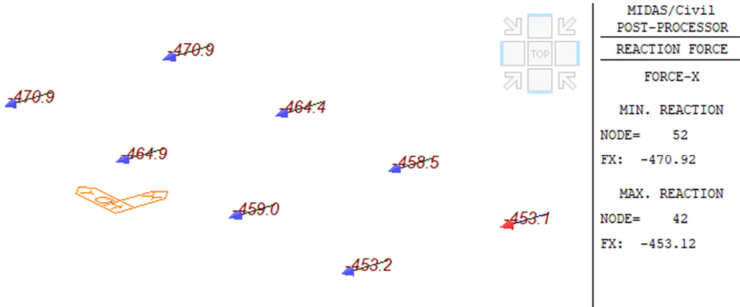
Figura 21 – Reazioni in direzione longitudinale
