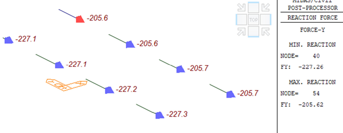
Figura 22 – Reazioni in direzione trasversale
