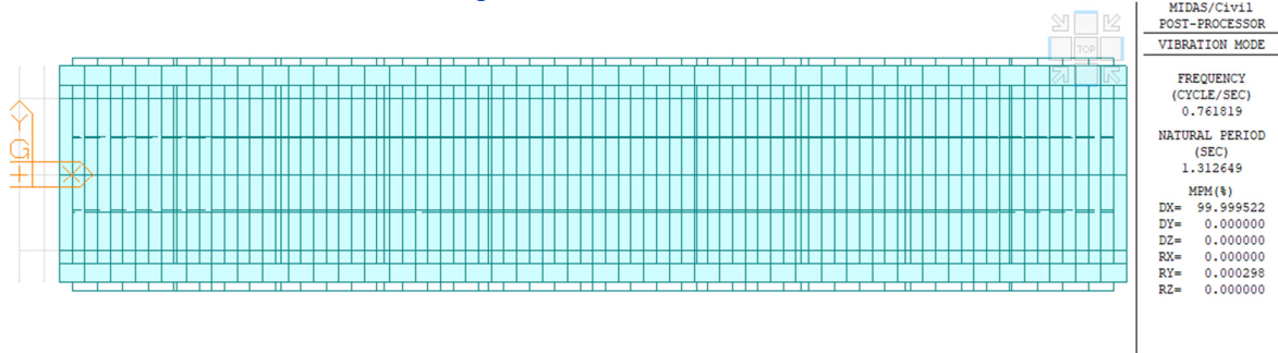
Figura 37 – Secondo modo di vibrazione
