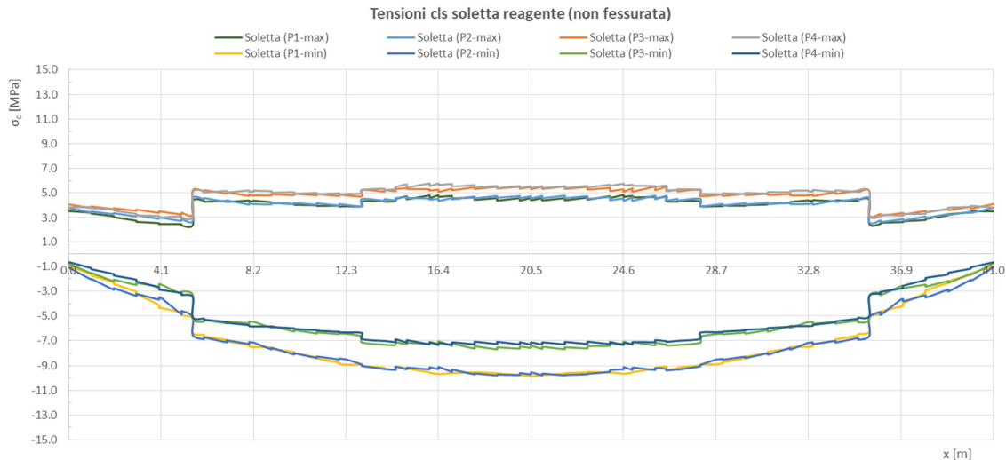
Figura 46 – Tensioni nella soletta nelle zone a calcestruzzo reagente (cls non fessurato)
