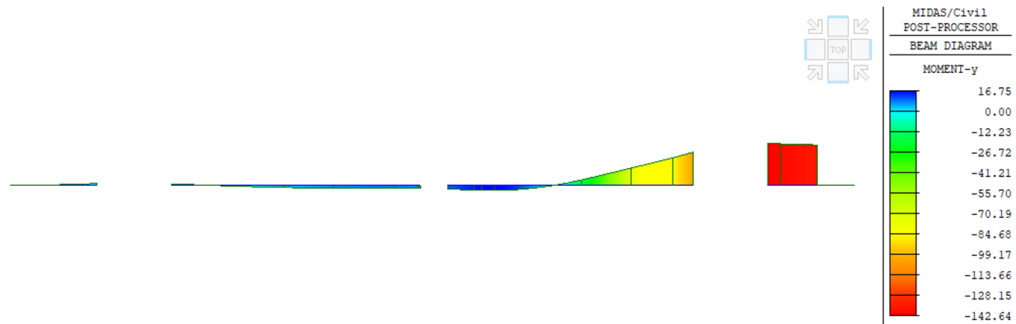
Figura 67 – Involuppo SLU-E – Momento flettente
