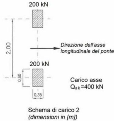
Figura 8 – Schema di carico 2
