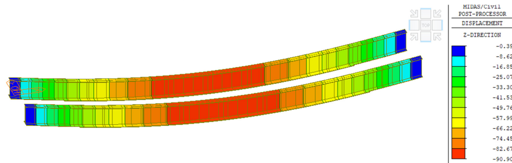
Figura 21 – G1.1+G1.2 – Spostamenti verticali D_Z
