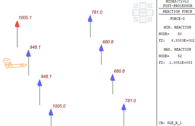
Figura 26 – Reazioni verticali
