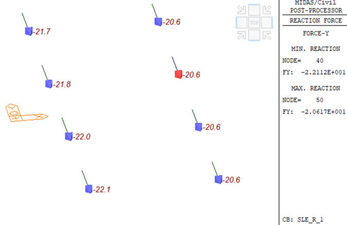
Figura 25 – Reazioni in direzione trasversale
