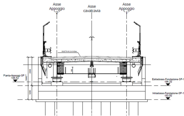
Figura 2 – Sezioni trasversali spalle
