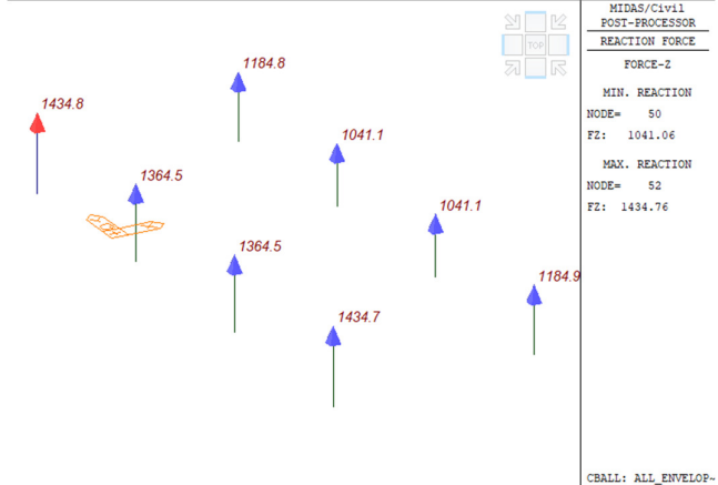
Figura 23 – Reazioni verticali
