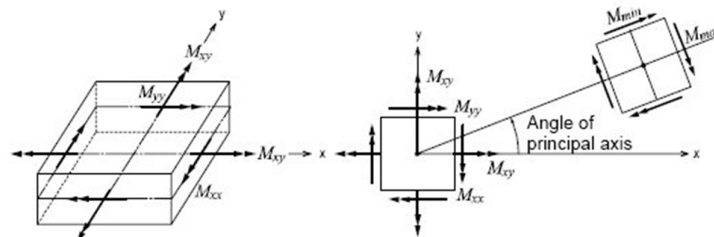
Figura 8 – Momenti negli elementi piani
