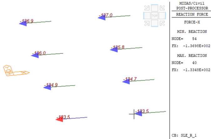
Figura 24 – Reazioni in direzione longitudinale
