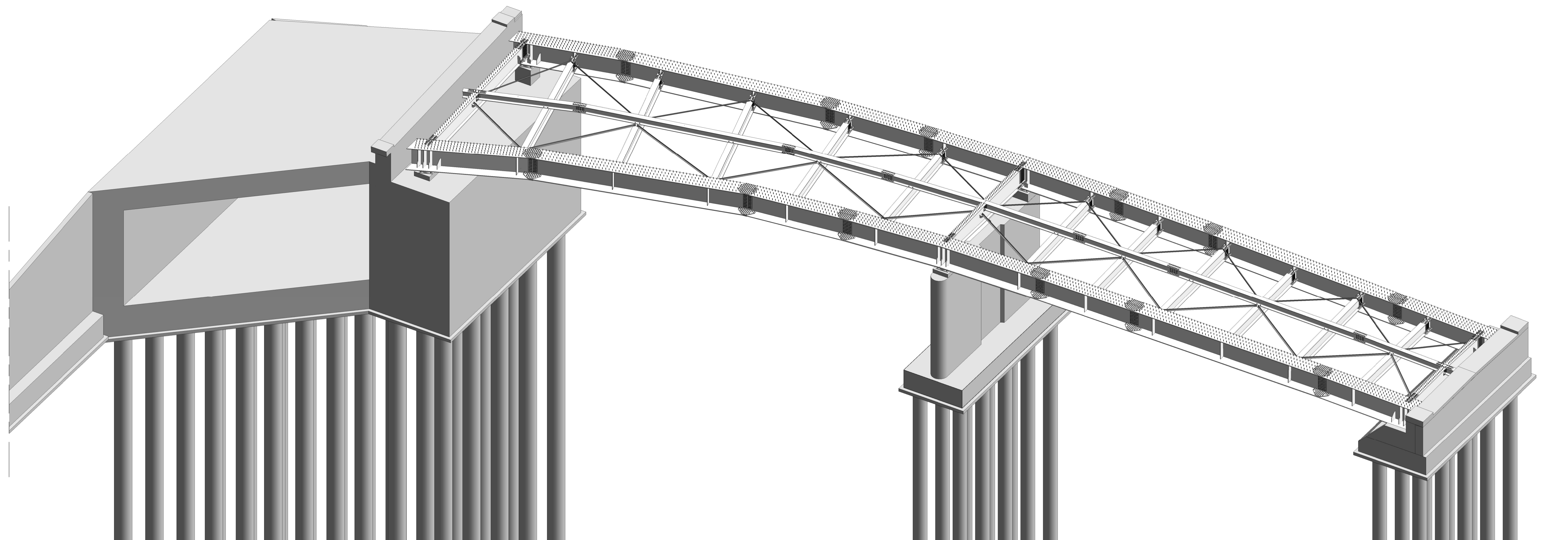
1 3D-Impalcato in acciaio
