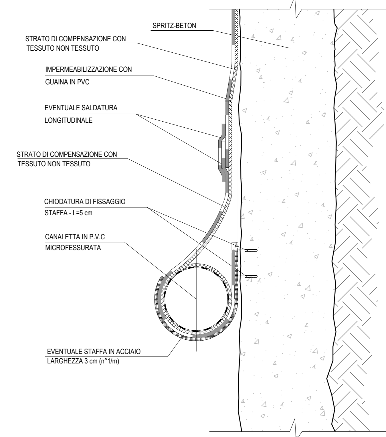
PARTICOLARE RISVOLTO IMPERMEABILIZZAZIONE SCALA 1:5
