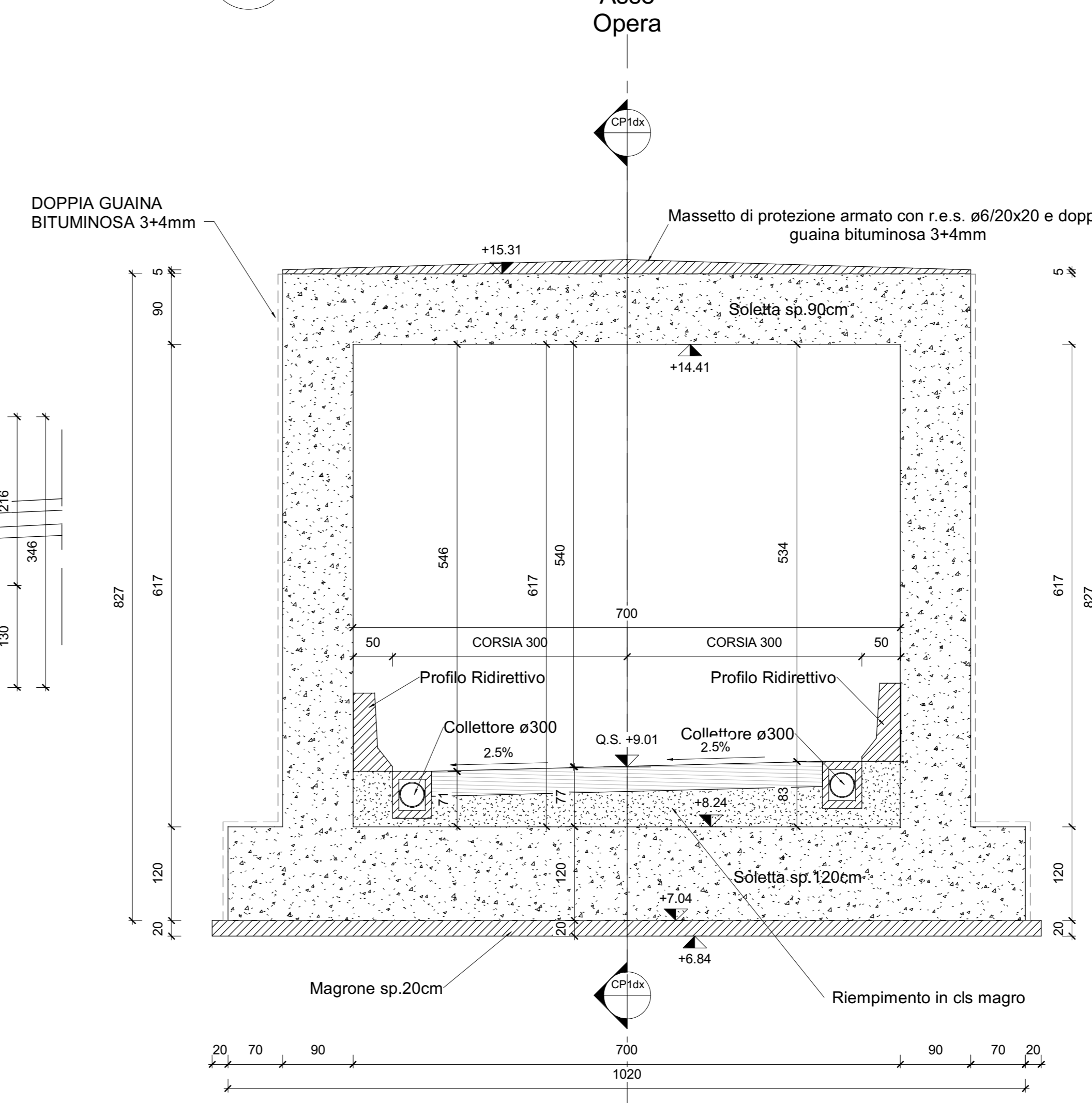
Sezione Trasversale Sottovia 1° fase - Carpenteria
