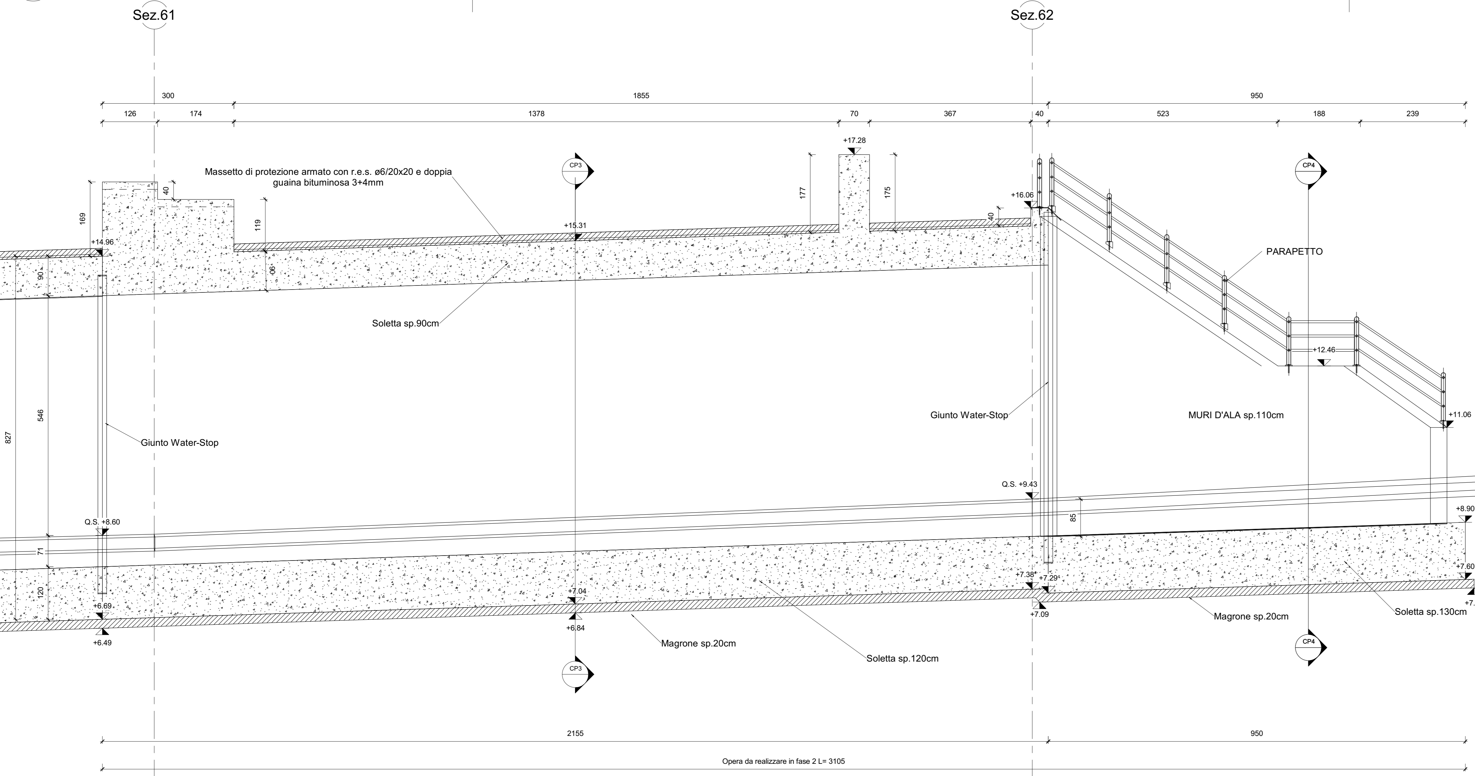
Sezione Longitudinale Sottovia - Carpenteria - sx
