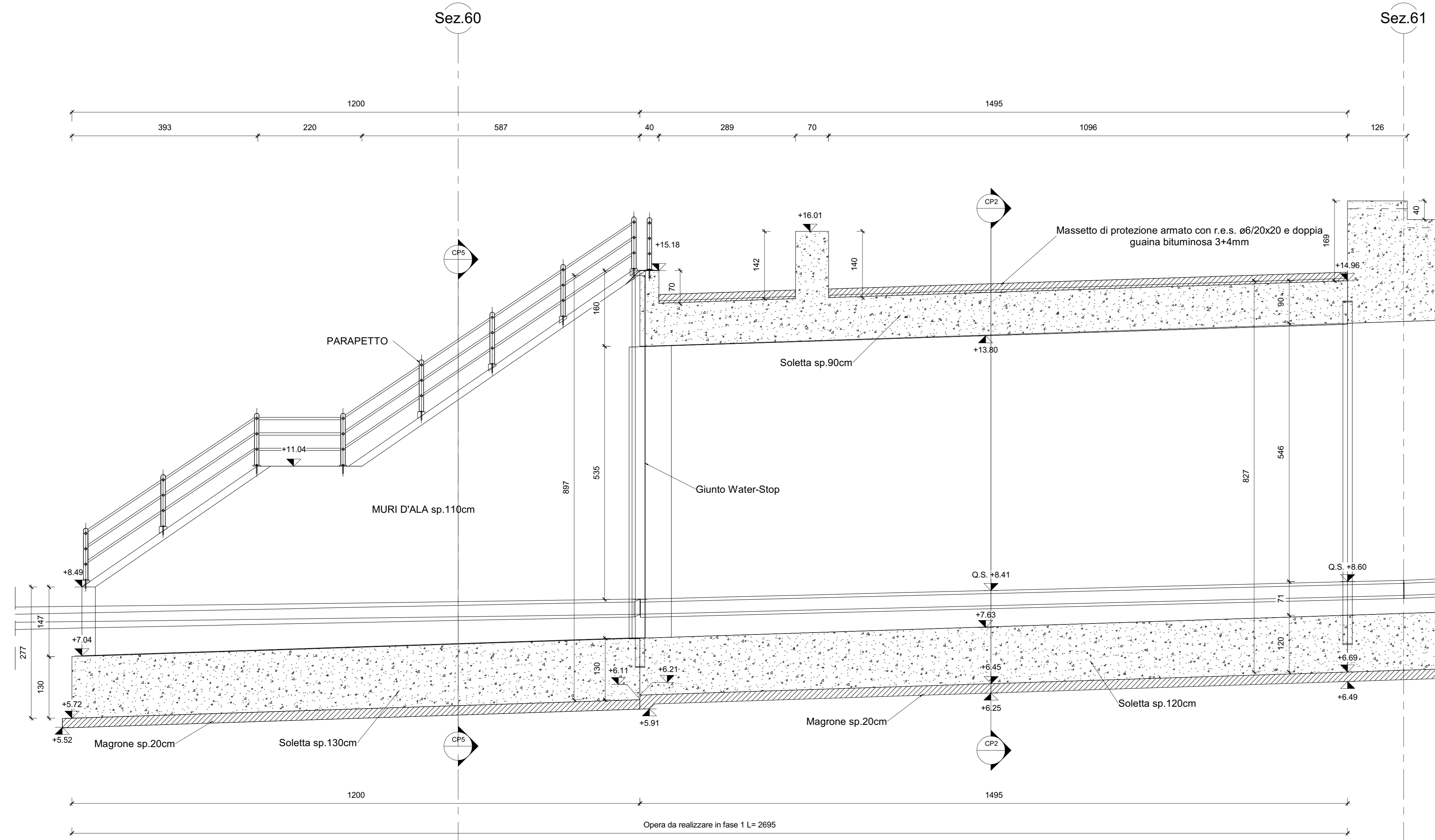
Sezione Longitudinale Sottovia - Carpenteria - sx
