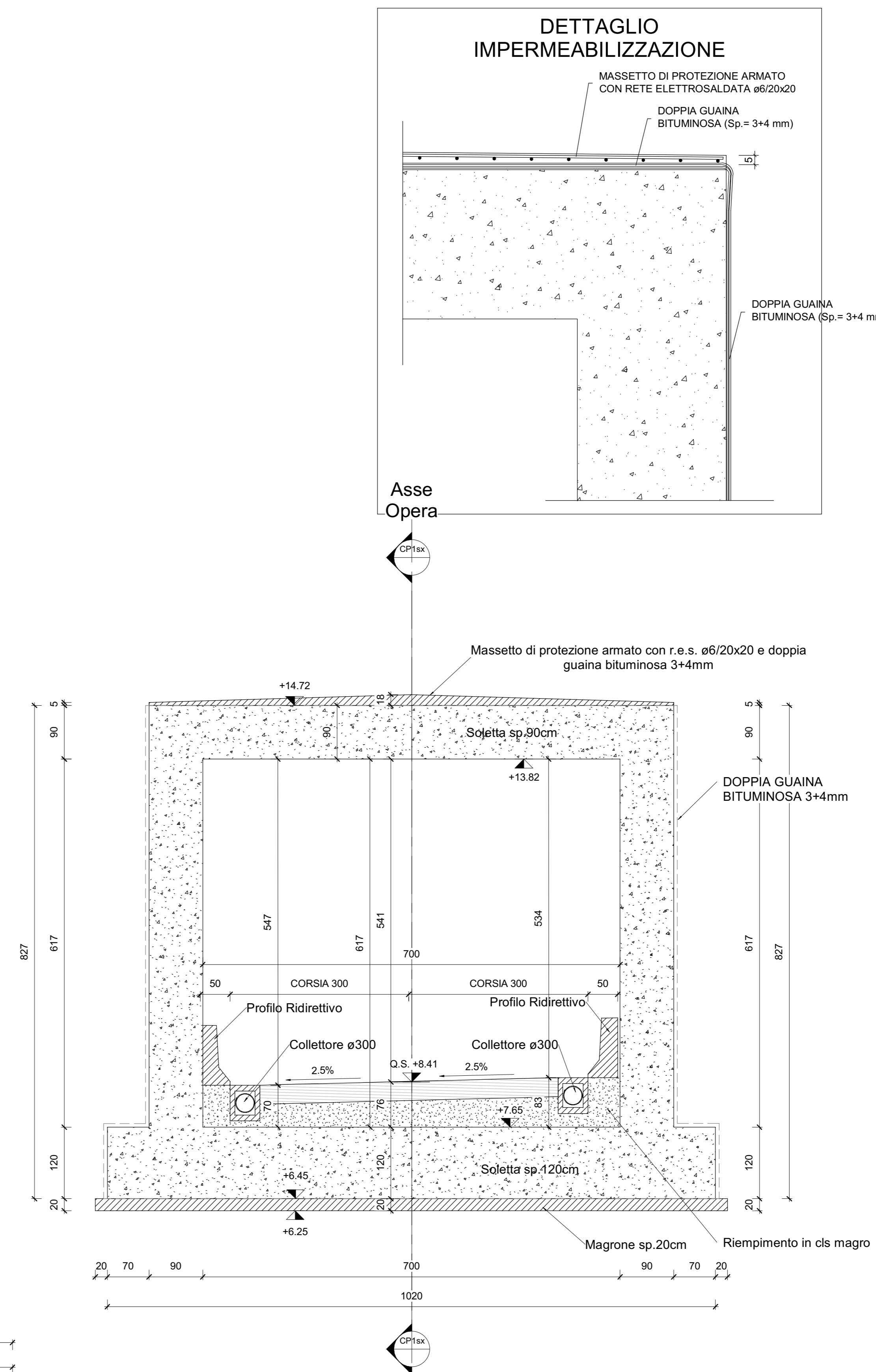
Sezione Trasversale Sottovia 1° fase - Carpenteria
