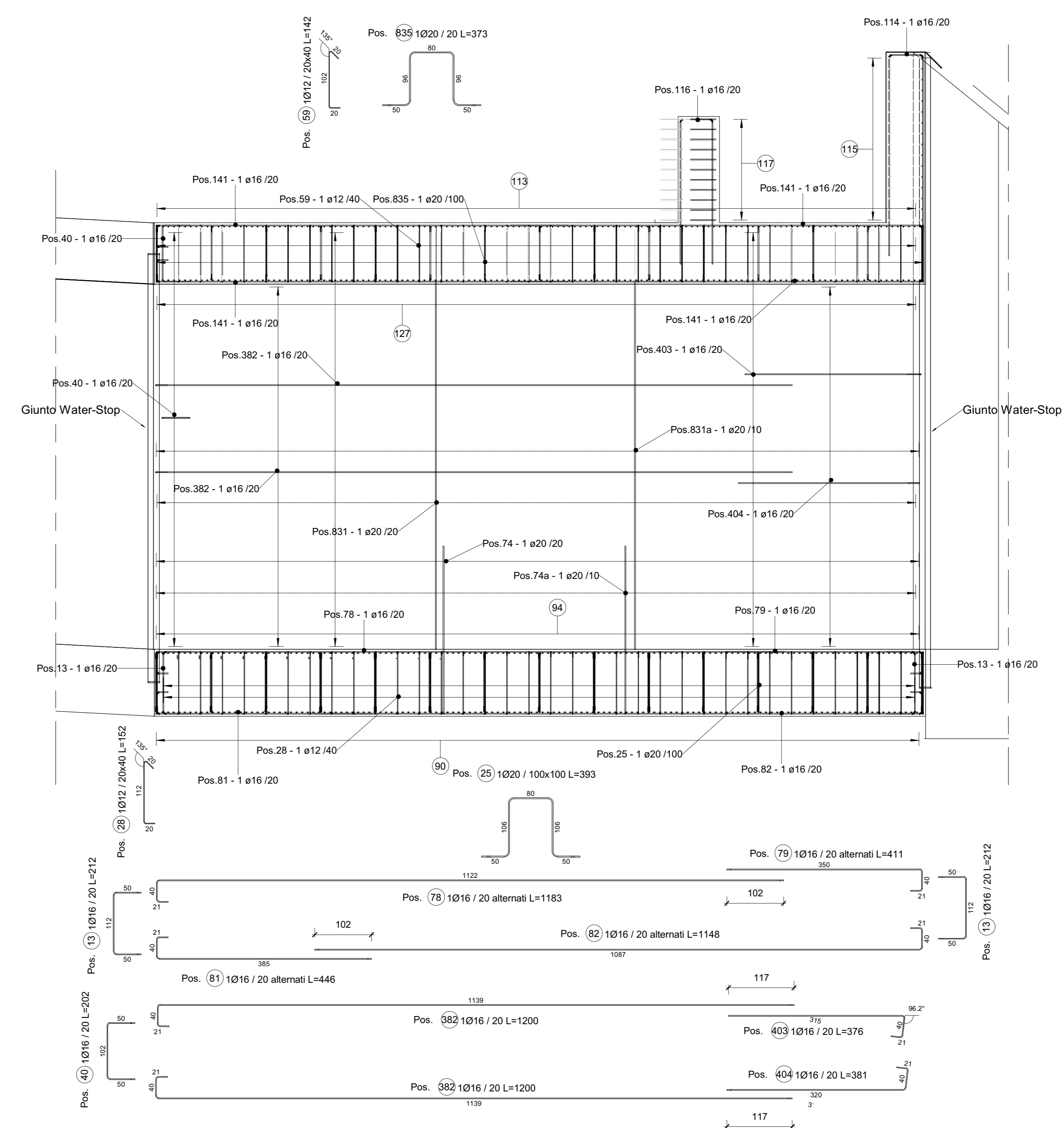
AR6 Sezione Longitudinale Sottovia 2° fase - Armatura 1 : 50
