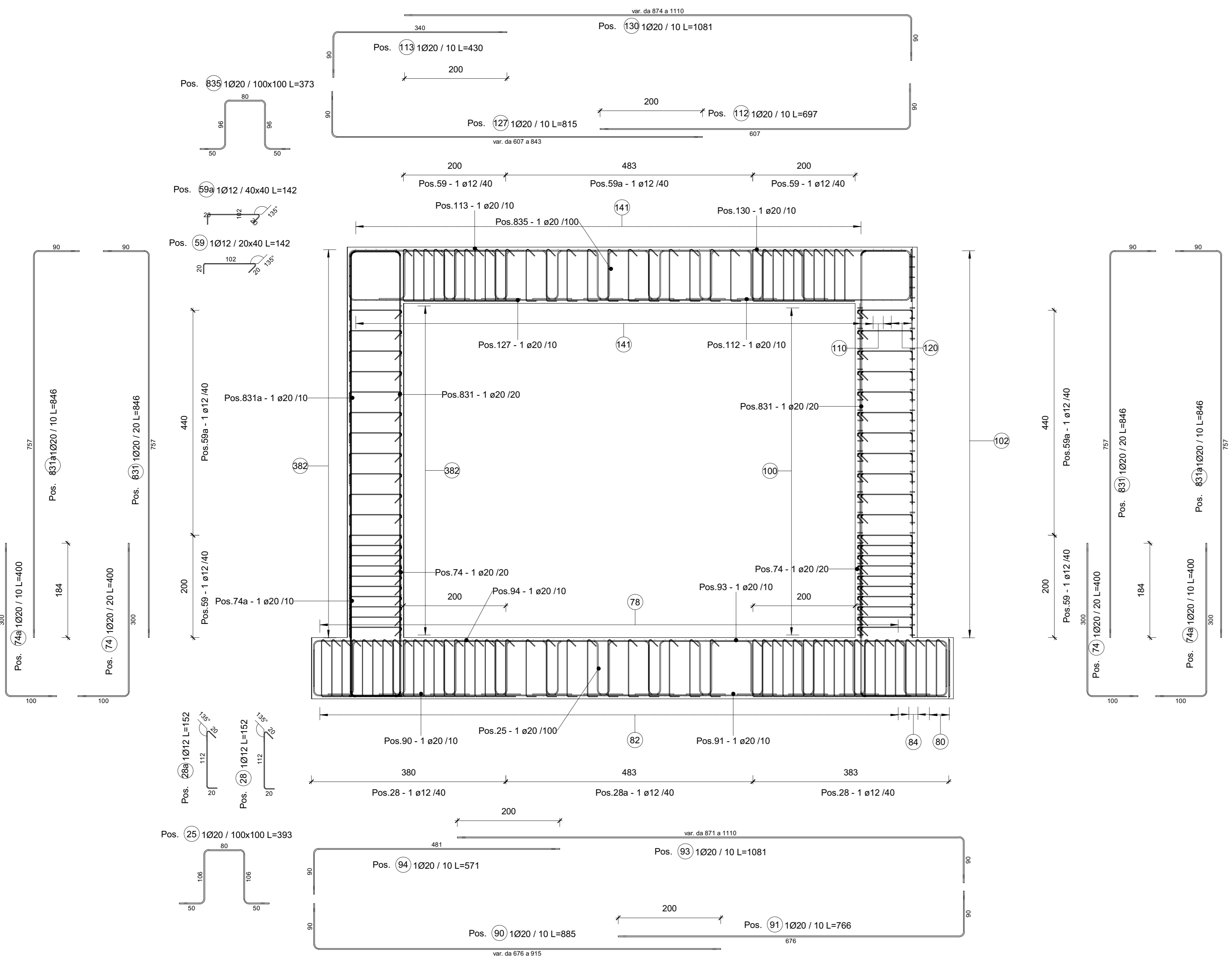
AR5 Sezione Trasversale Sottovia 2° fase - Armatura 1 : 50
