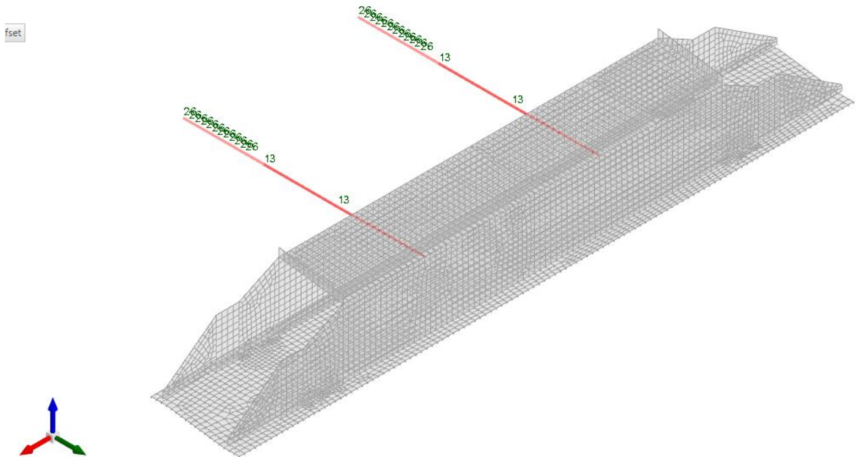
Figura 7 - Condizione frenatura
