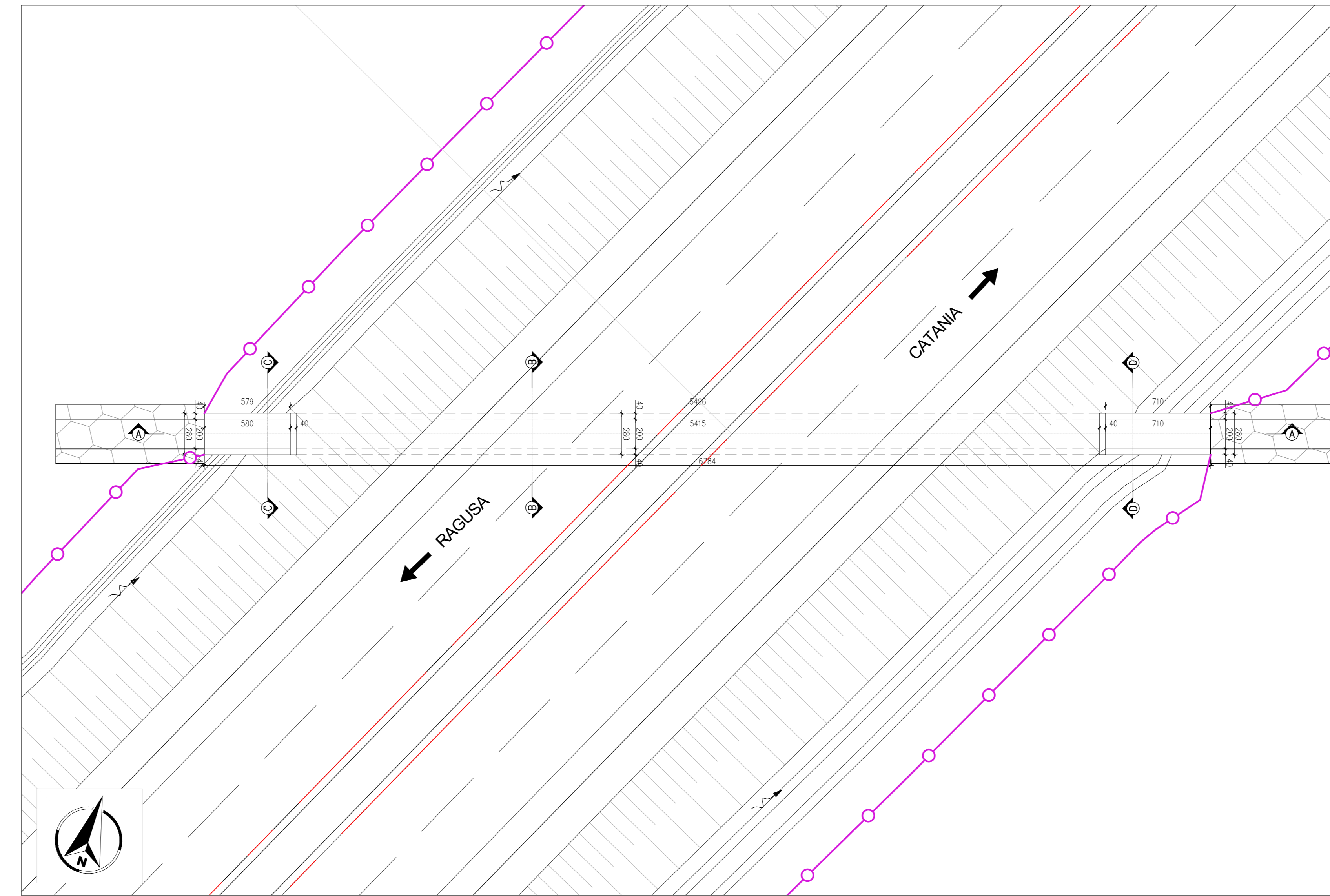
PLANIMETRIA SCALA 1:200
